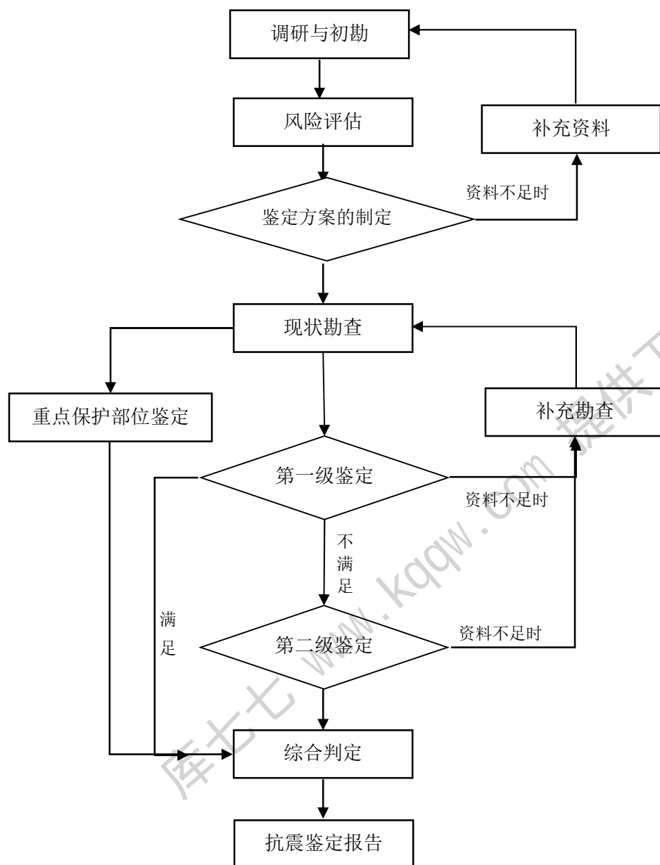
图1 文物建筑抗震鉴定程序
