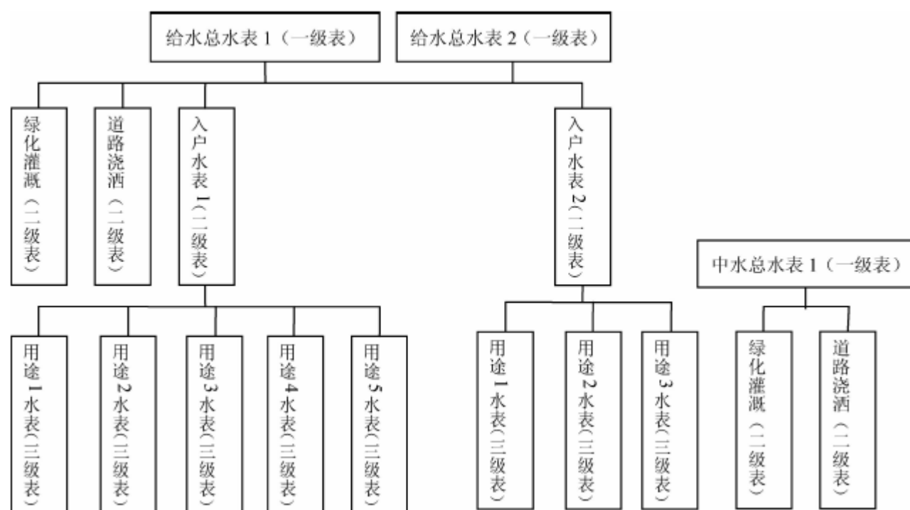
图 6.1.2 水表分级示意图
