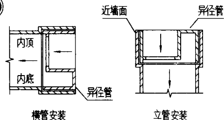
异径管大样
