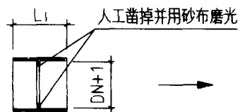
有挡管箍
