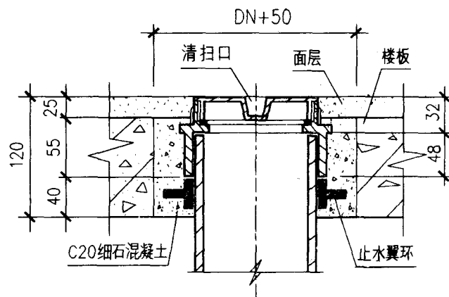
清扫口大样
