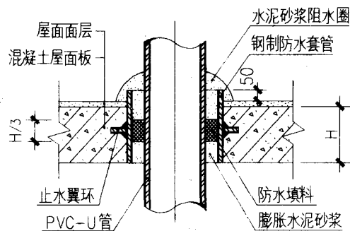
穿屋面 (I 型)
