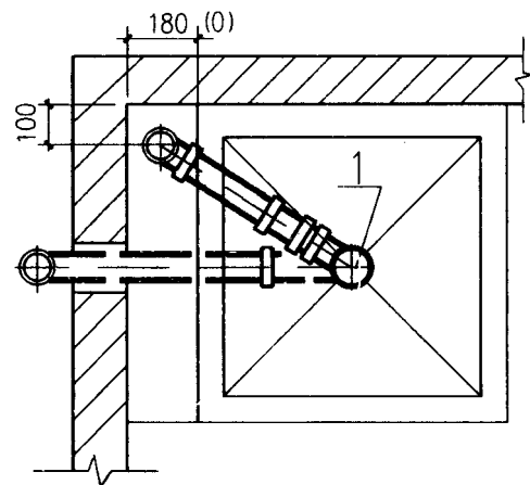
洗涤池平面
