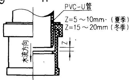
I型伸缩节大样
