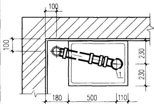
洗涤盆平面
