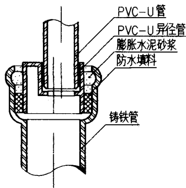
异径管
