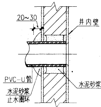
穿检查井壁
