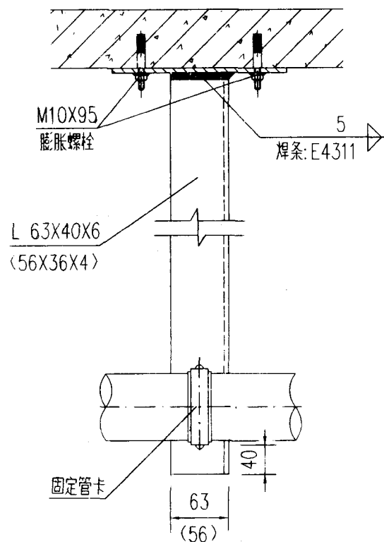
立面
