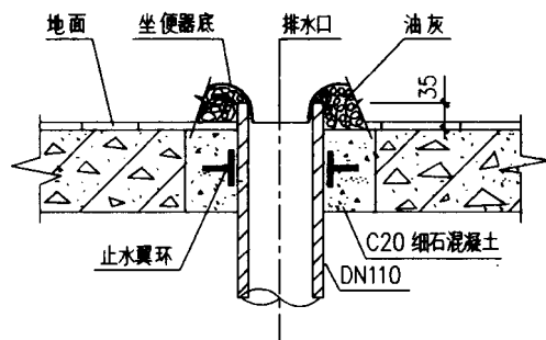
A 节点
