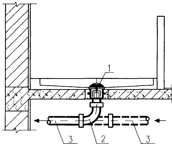
立面图
