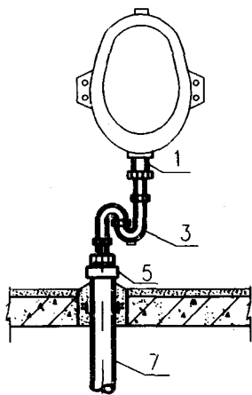
挂式正立面
