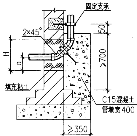
墙基留洞
