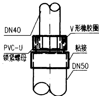
转换接头 I
