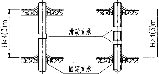
图 1 立管支承示意
