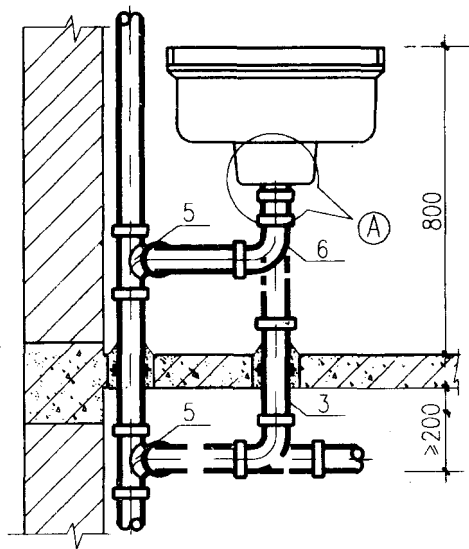
化验盆正立面
