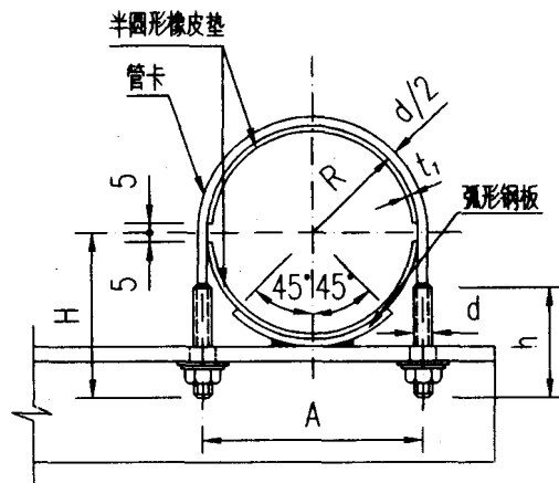
立面
