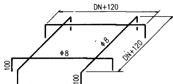
管加强钢筋
