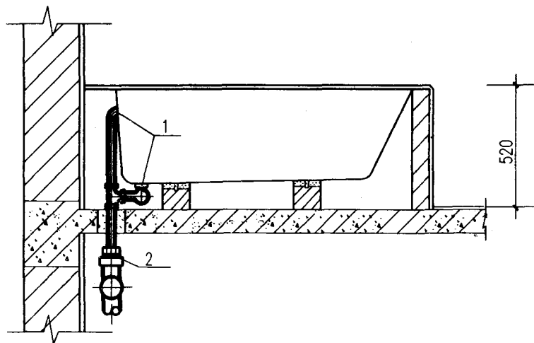
1-1剖面
