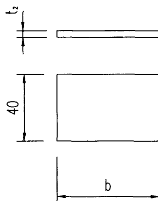
弧形钢板展开
