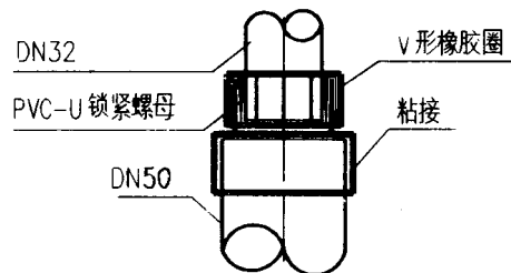
转换接头
