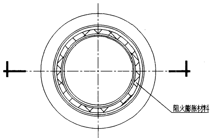
阻火圈平剖面
