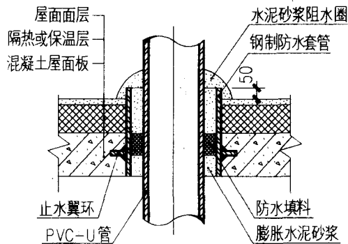
穿屋面 (II 型)
