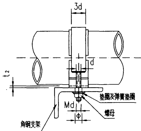
侧面
