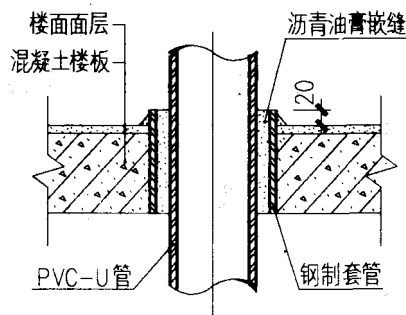
穿楼面 (II 型)
