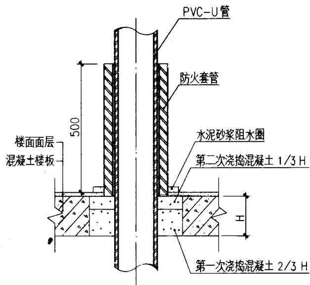
I 型立管防火套管
