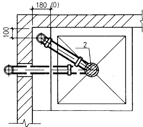
污水池平面
