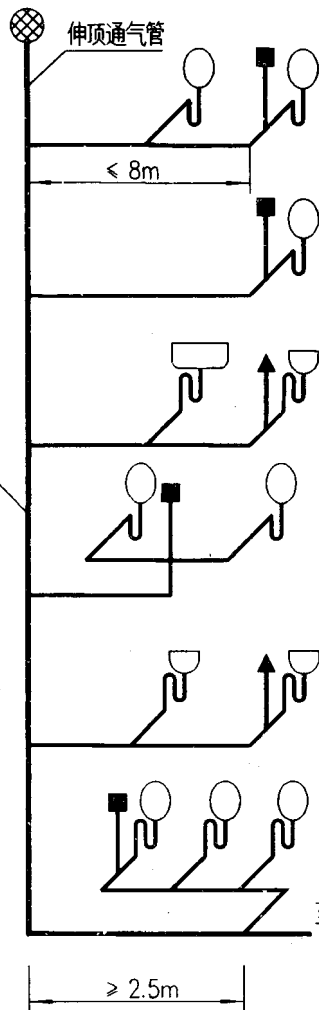
排水系统吸气阀安装图式 1 (用于 1~16 层建筑)
