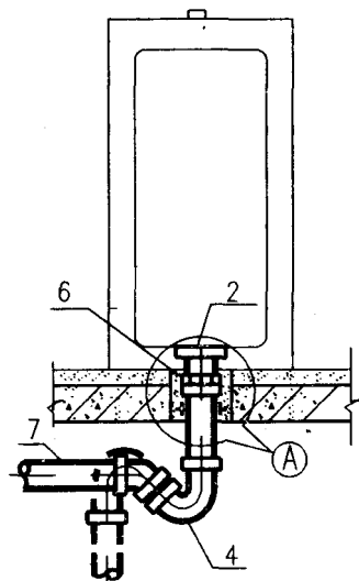
立式正立面
