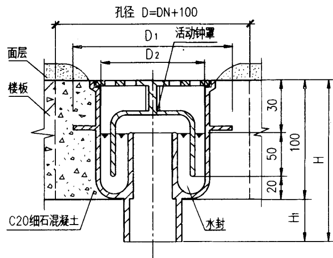
I 型地漏
