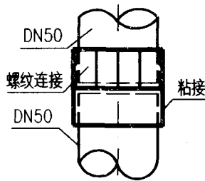
转换接头 II
