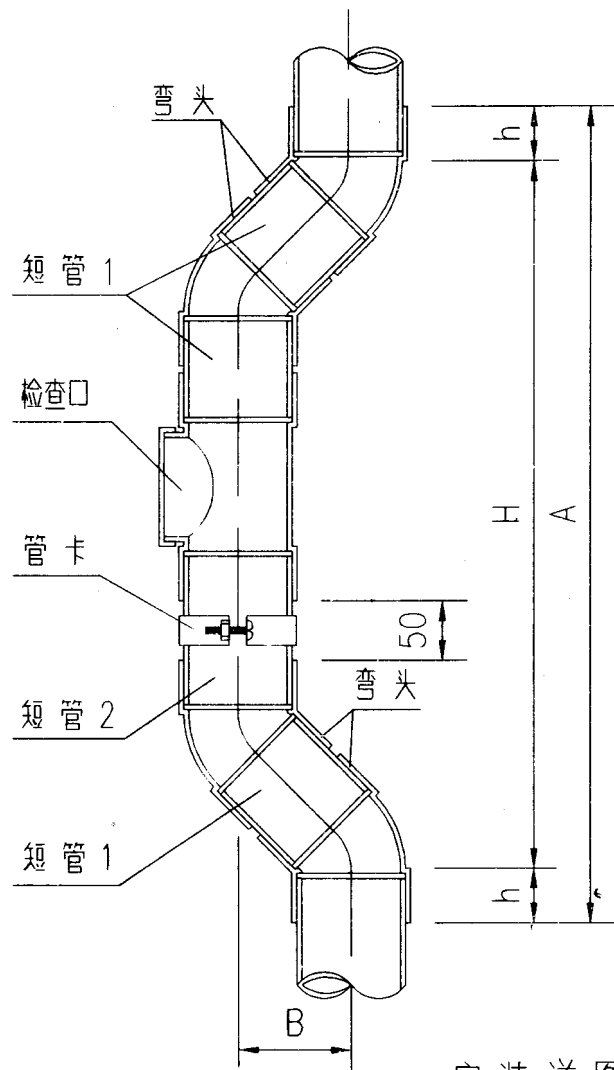
安装详图
