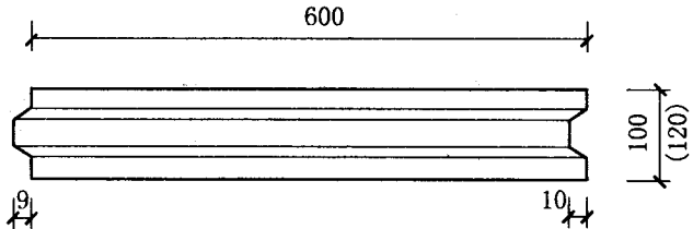
实心砌块端面示意图
