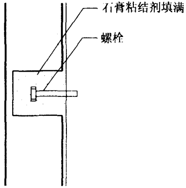
2 隔墙埋螺栓安装图
