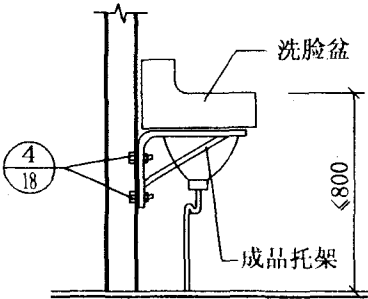
1-1 剖面图
