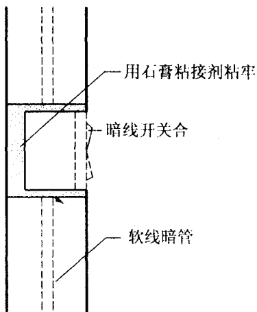
3 暗线开关安装
