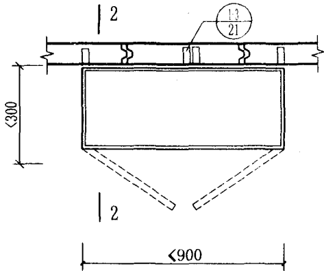
吊柜平面
