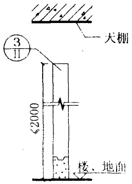
隔断墙
