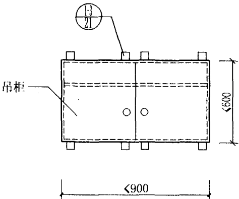
吊柜立面
