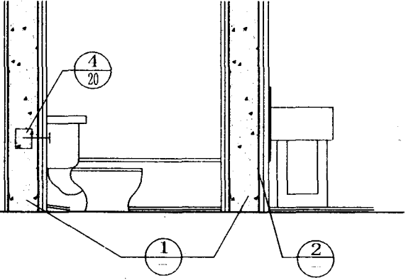
1-1 剖面图
