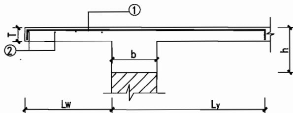
①~② 平衡板式平板挑檐
