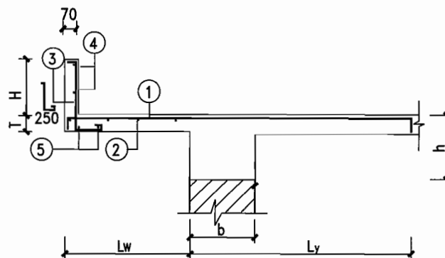
⑤~⑩ 平衡板式直翻沿挑檐
