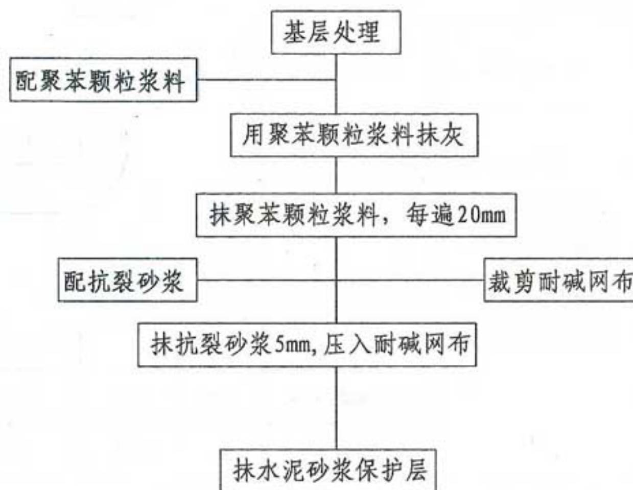
施工流程图
