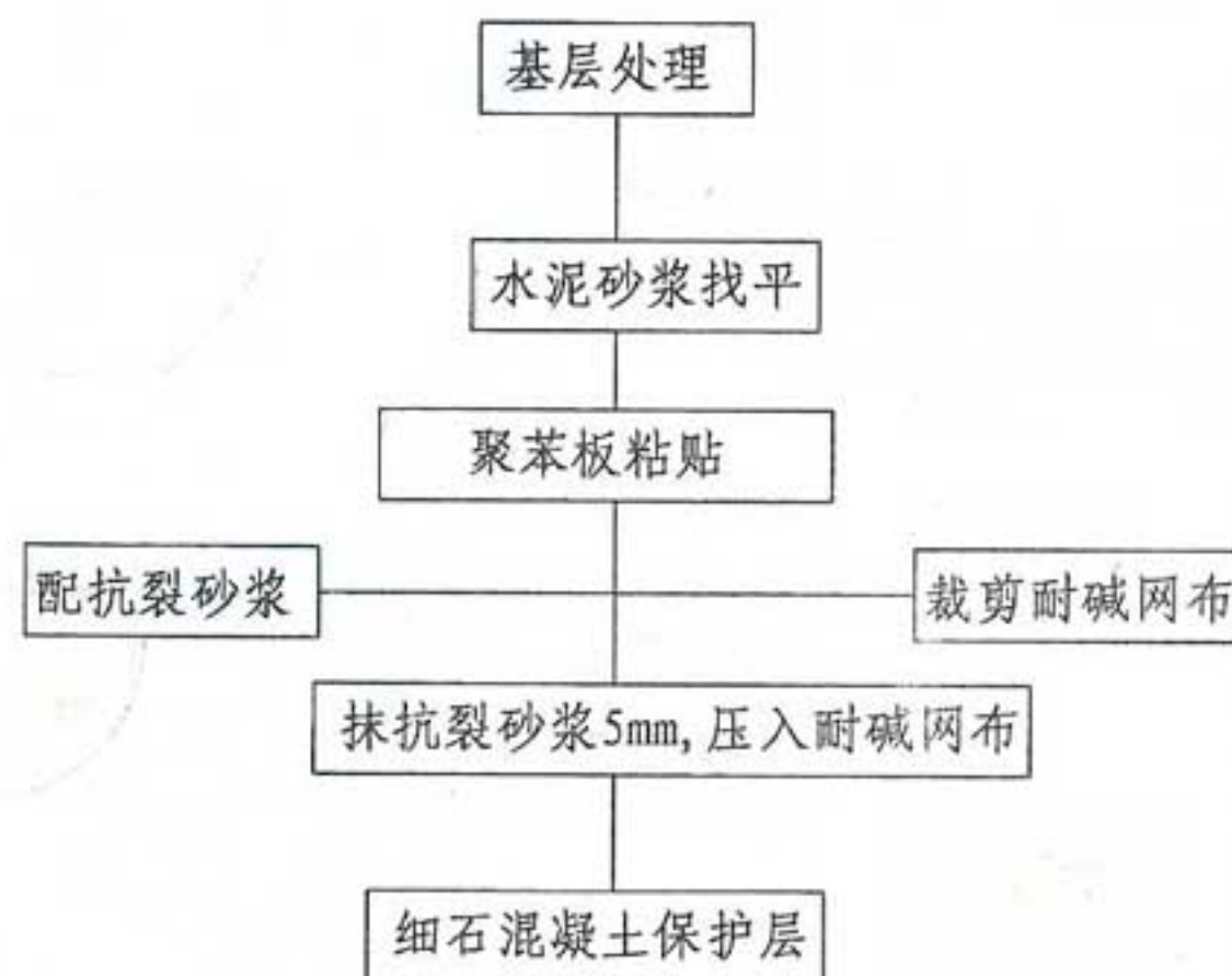
施工流程图
