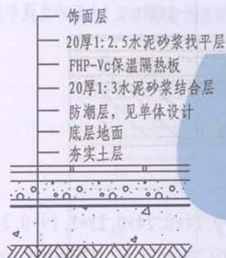
2 底层地面
