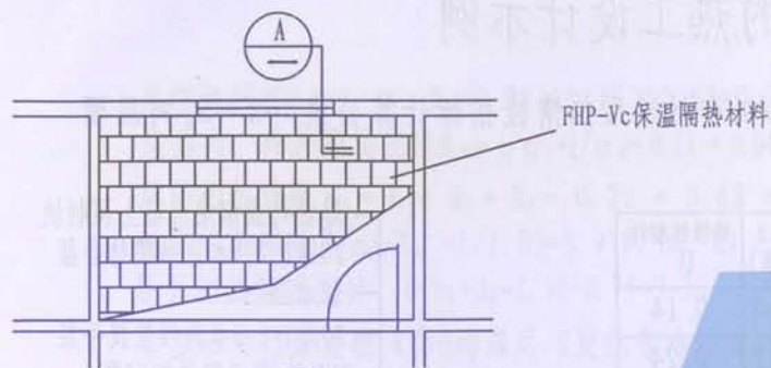
1 保温隔热板铺装图
