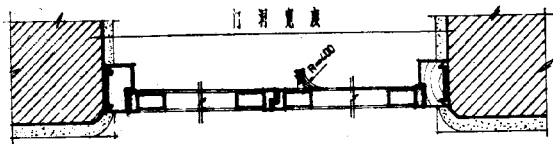
大、小扇门剖面图
