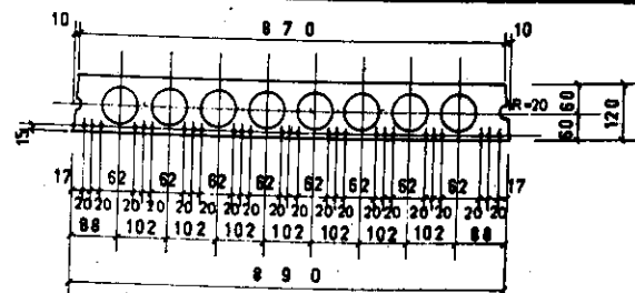
3 型板配筋图
