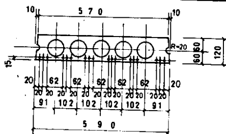
2型板配筋图
