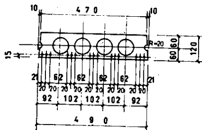
一、型板配筋圖
