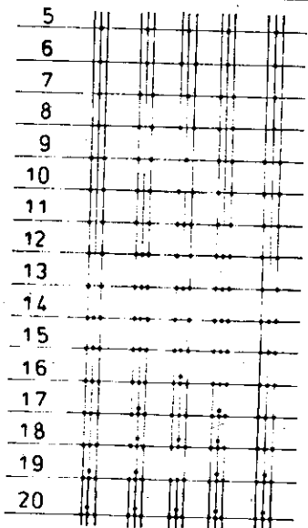
一、型板配筋圖
