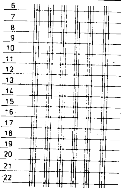
2型板配筋图
