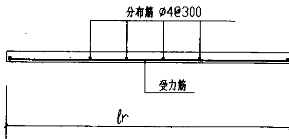
1-1 剖面图
