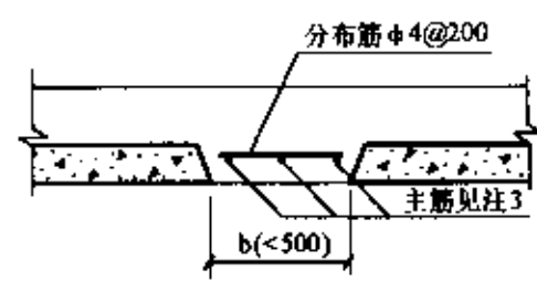
补空板示意图
