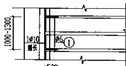
1-1 用于现浇板
