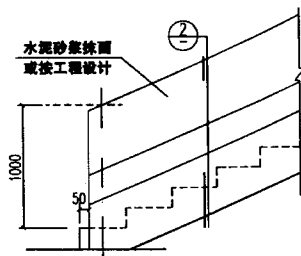
混凝土栏杆 2 立面图
