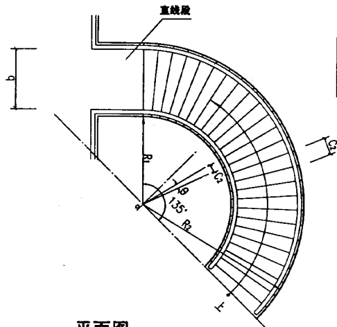
平面图
