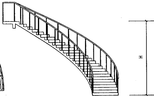
立面图
