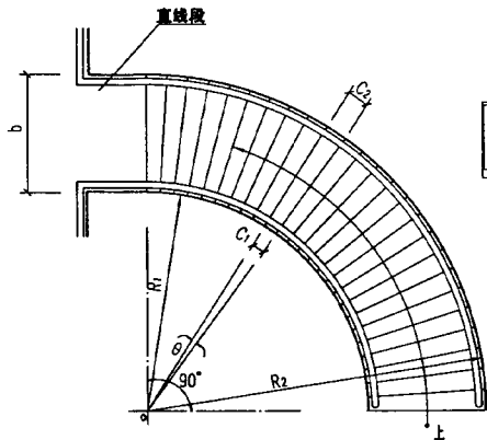
平面图
