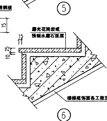
面层花饰分格, 详图
