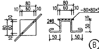
楼梯顶端栏杆 详图
