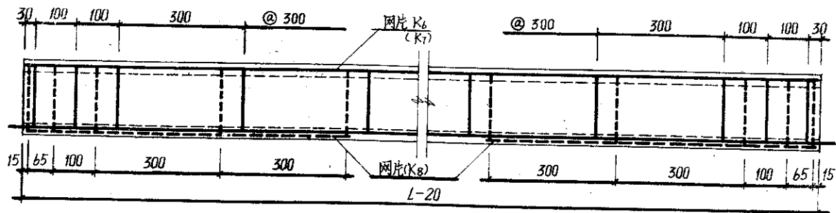
2型板详图
