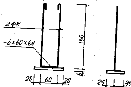
板 底 予 埋 件
