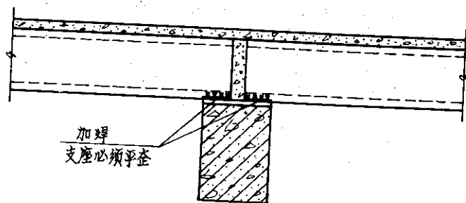
梁 或 内 埠 搁 置 构 造
