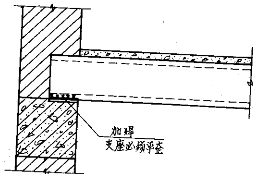
外 埠 搁 置 构 造
