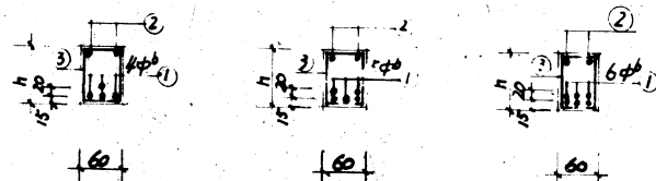
预应力钢筋混凝土檩条的三种断面配筋情况
