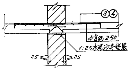
连续板中间支座构造
