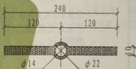
Ⓐ 可卸式橡胶止水带
