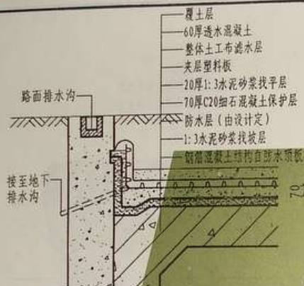
① 边沿围护排水
