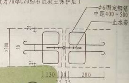
③ 止水带固定钢筋
