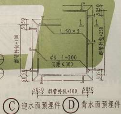
群管穿墙防水构造
