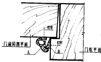
巧力碰珠门上安装平面位置示意
