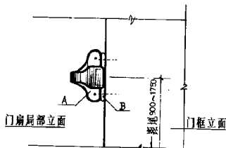
巧力碰珠门上安装立面示意
