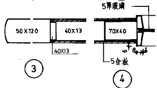
11 骨架立面 (典型立面3、8号门)
