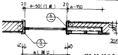
(三) 暗装推拉门平面
