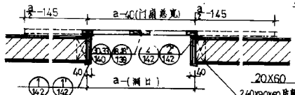
双扇: (五) 双扇明装推拉门平面
