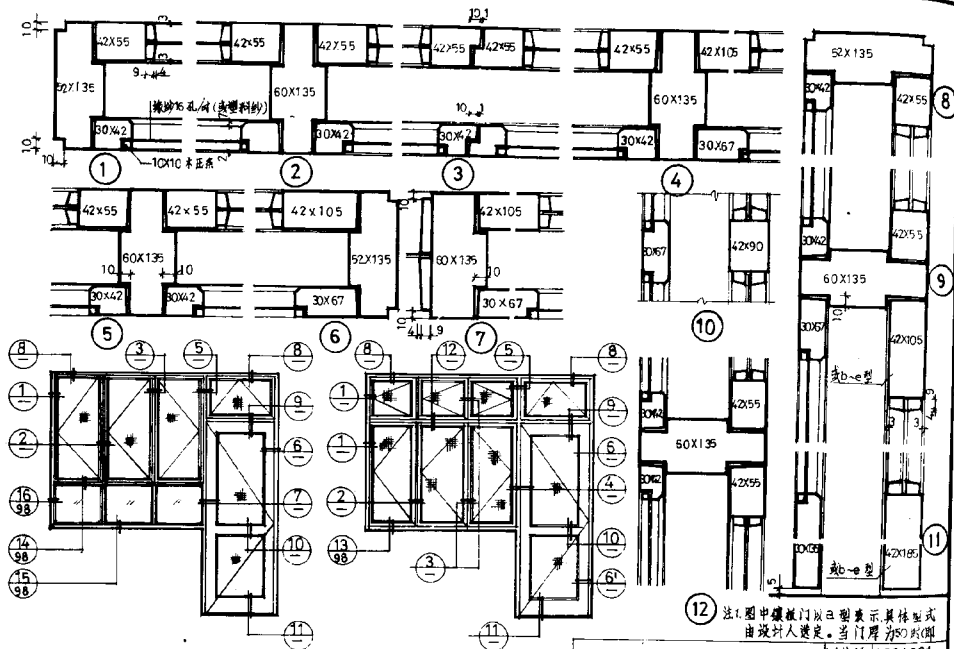
M4 连窗门帘纱扇典型立、剖面
