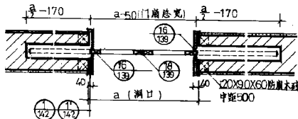
(四) 双扇暗装推拉门平面
