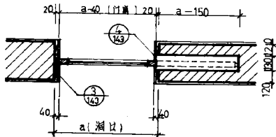
(一) 暗装推拉门平面
