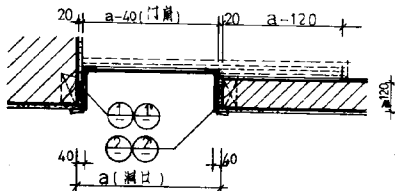
(二) 明装推拉门平面
