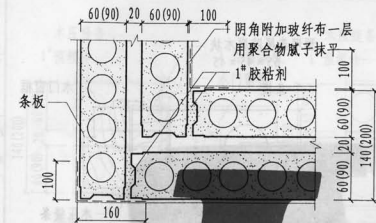
① 双层条板直角连接
