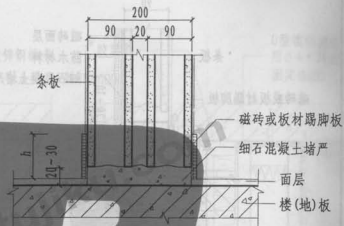
② 双层条板与楼地面连接(二)
