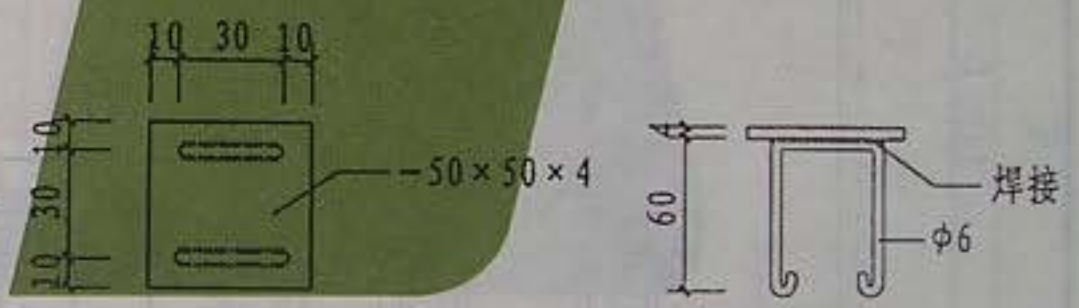
M-1预埋铁件
