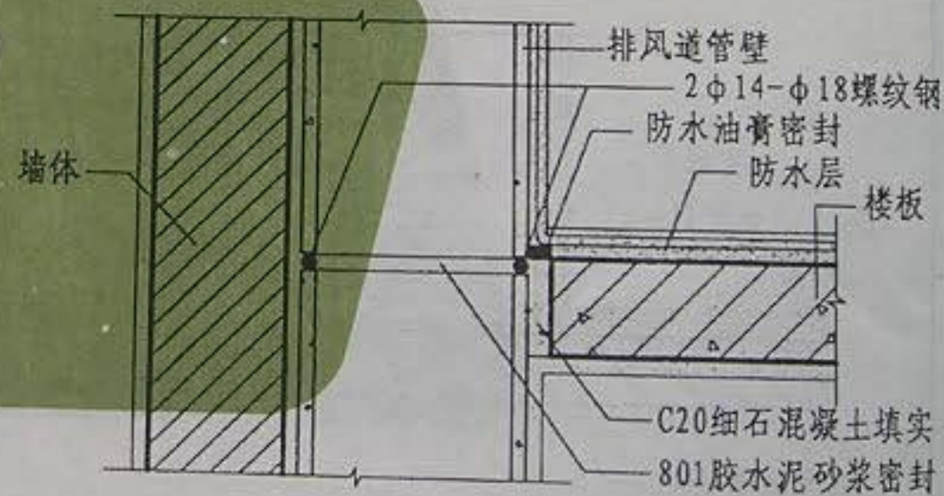
② 排风道承托示意 (用于下沉式厨房、卫生间)
