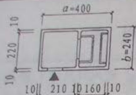
编号:1 型号: PCZI6 排风道: a \times b = 400 \times 240 预留洞: a_1 \times b_1 = 450 \times 290
