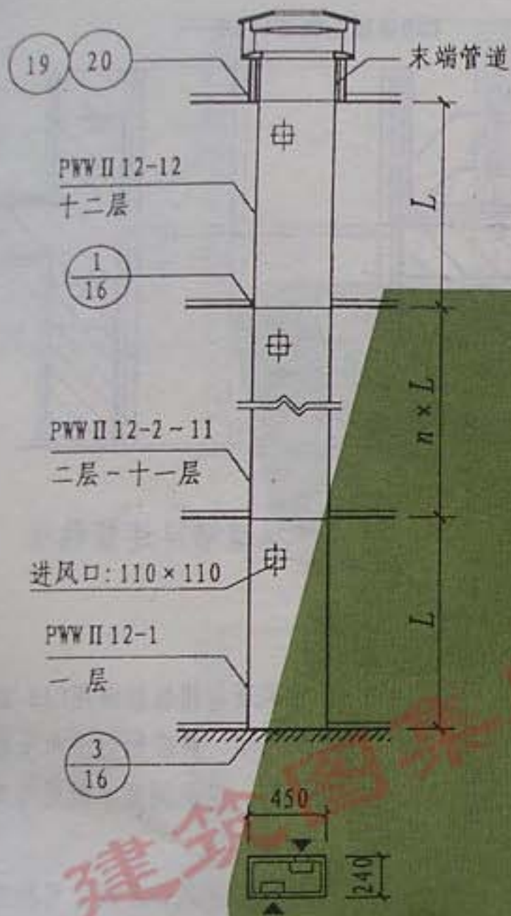
PWW II 12 型系统组装示意图
