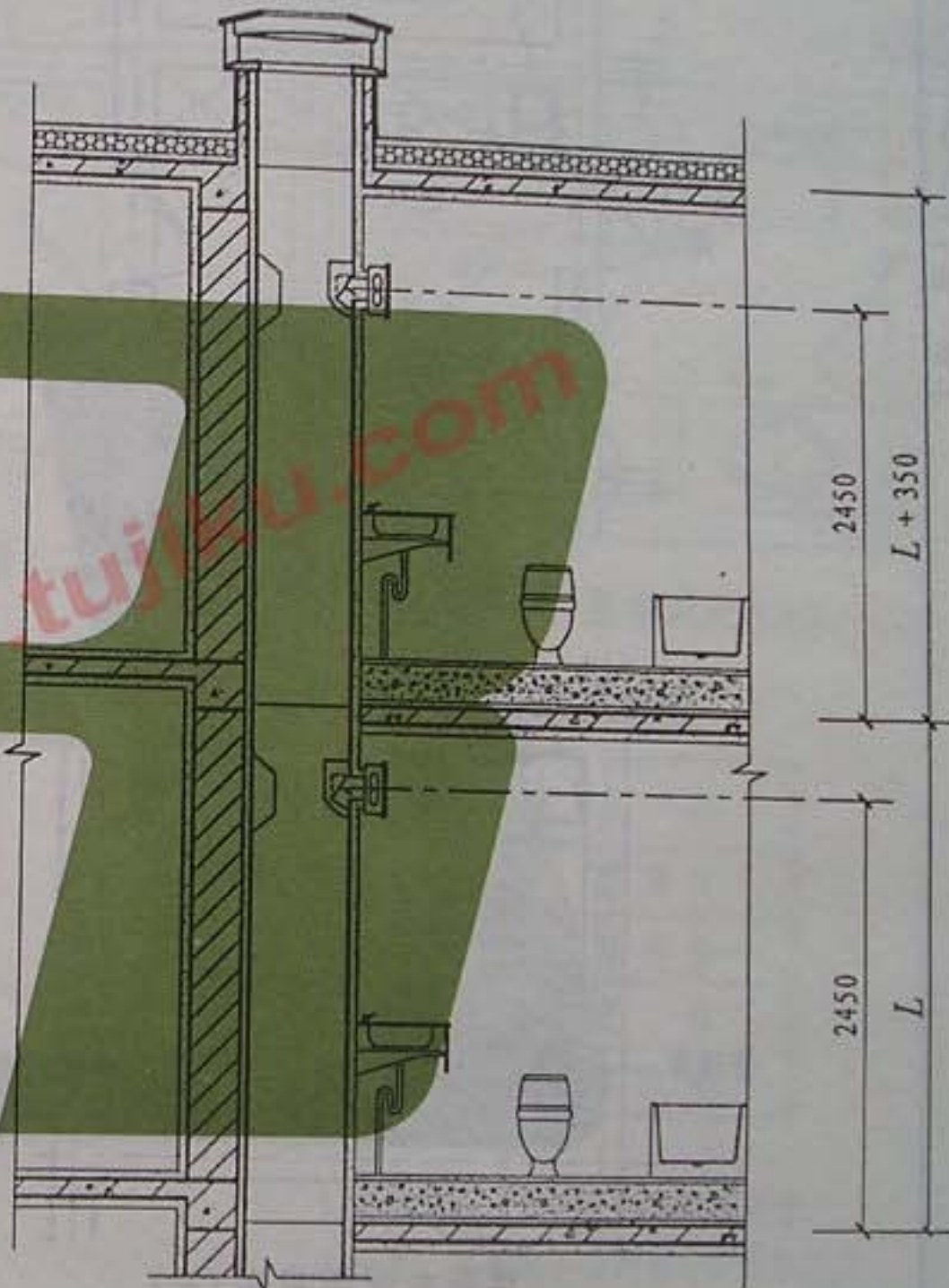
卫生间(下沉式)排风道安装示意图
