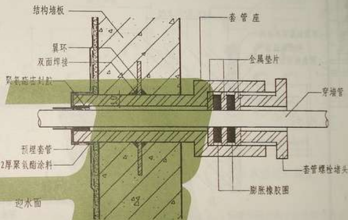
② 单管橡胶圈密封法
