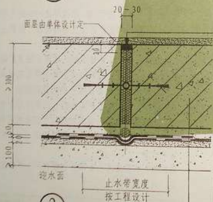
② 底板
