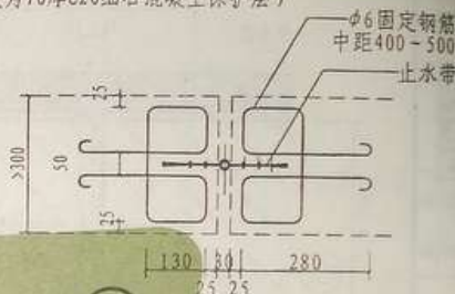
③ 止水带固定钢筋
