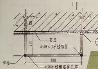
① 不锈钢爬梯节点详图
