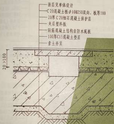
① 底板面架空防排水组合构造
