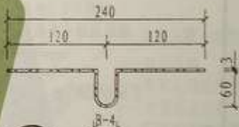
Ⓑ 金属止水带 B: 变形缝宽
