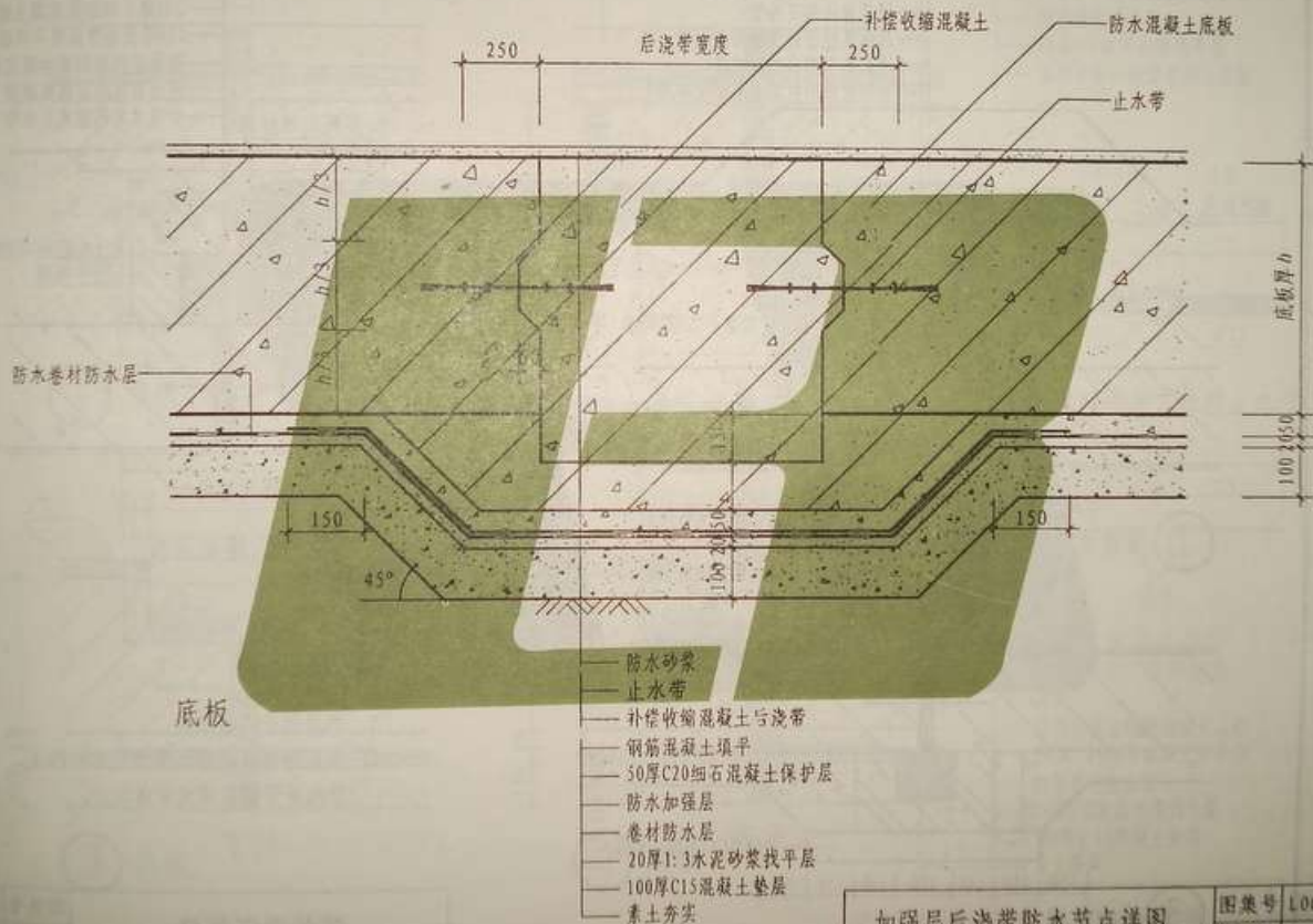
加强层后浇带防水节点详图
