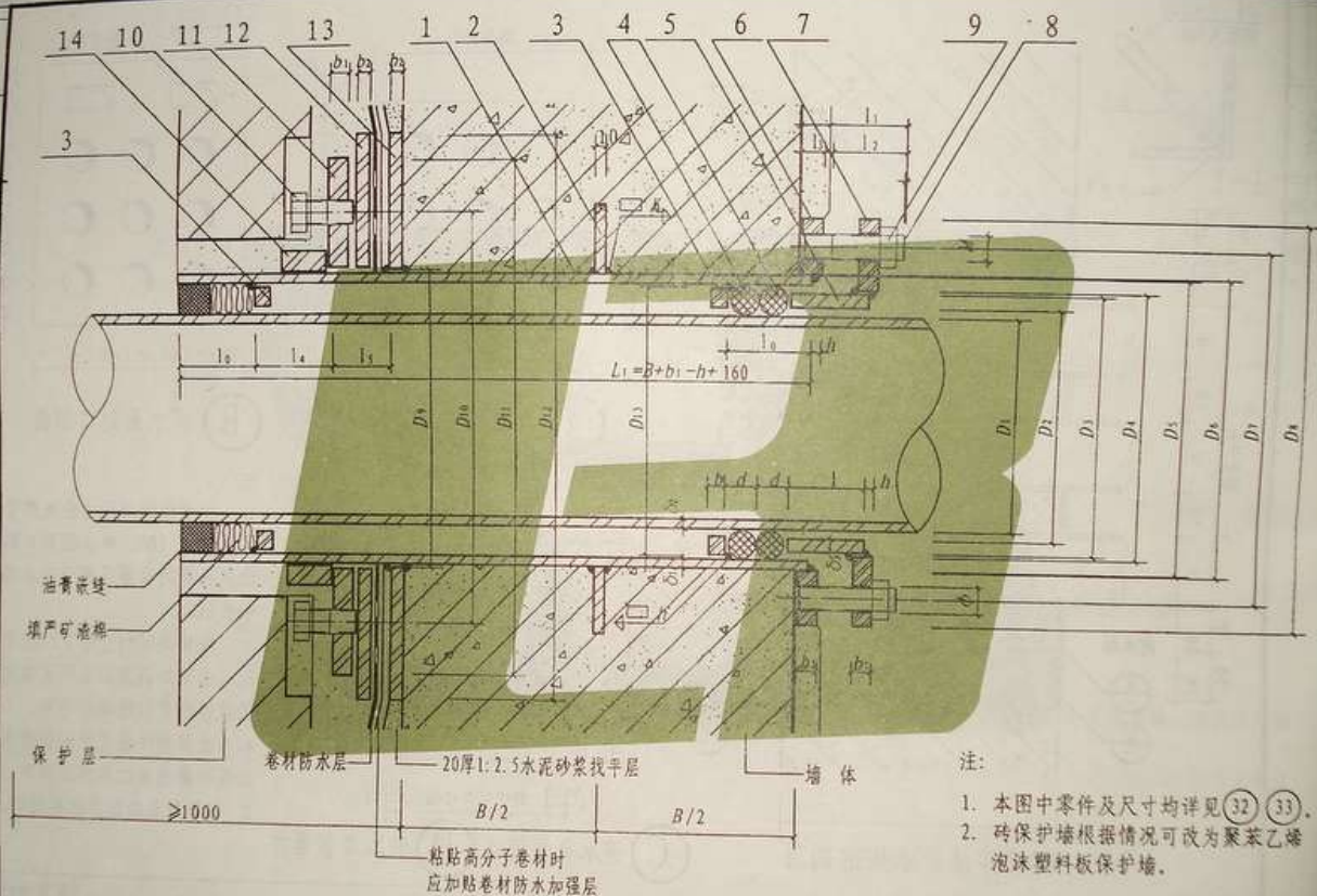
柔性防水穿墙套管(一)
