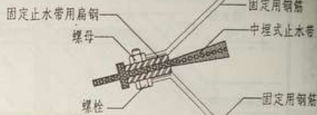
③ 止水带固定节点
