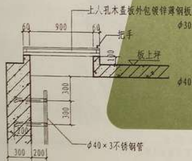
② 水池检修孔详图
