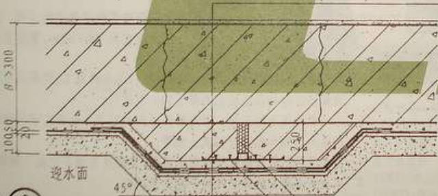
③ 底板
