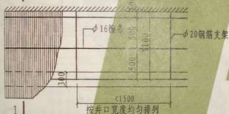
2 | ① 钢筋支架平面
