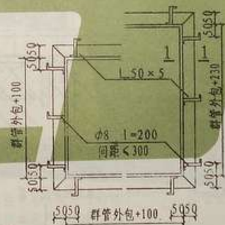
(C) 迎水面预埋件 (D) 背水面预埋件
