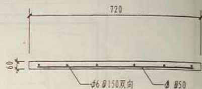
③ 预制混凝土盖板配筋
