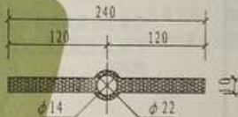
Ⓐ 可卸式橡胶止水带
