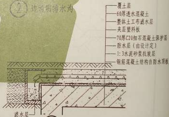
④ 边沿盲沟排水
