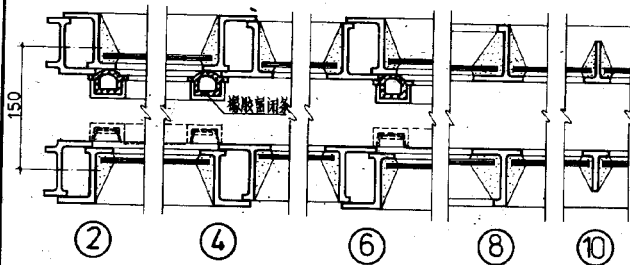
双层密封窗立面示意
