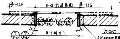
双扇: (五) 双扇明装推拉门平面
