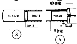
门骨架立面 (典型立面3、8号门)
