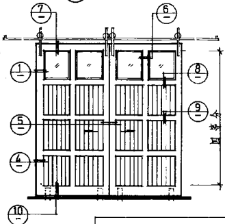
M8 推拉门典型立面及剖面
