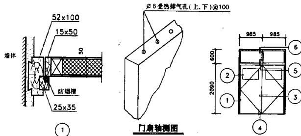
典型立面节点示意
