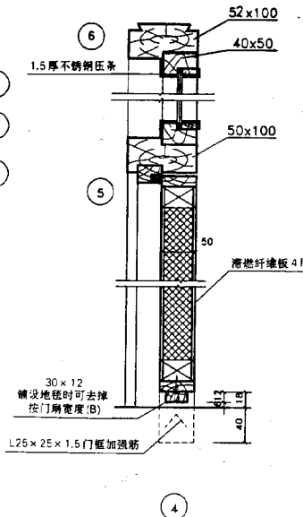
典型立面节点示意
