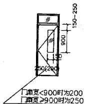
防火玻璃镶在门扇右(左)上角
