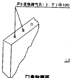
门扇轴测图
