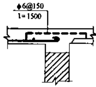
人孔板端部联接(二)
