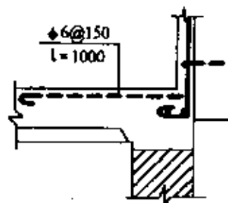
人孔板端部联接(一)
