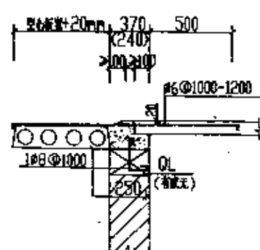
⑥ 屋盖
