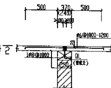
③ 屋盖
