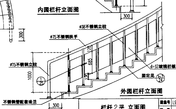
栏杆 2 平、立面图
