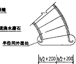
楼梯起步处理 2
