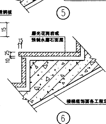
面层花饰分格 详图
