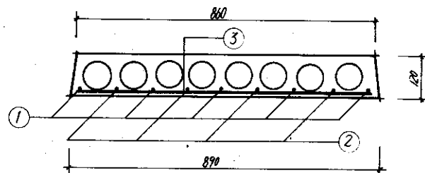
II—II 剖面
