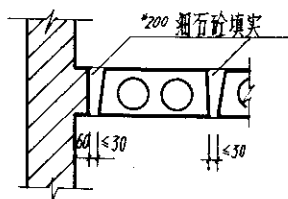
样挑砖做法
