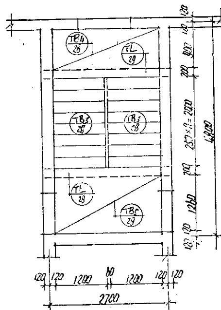
标准层平面
