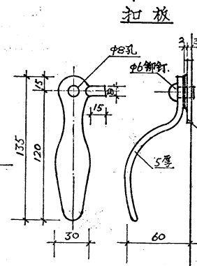
扳手
