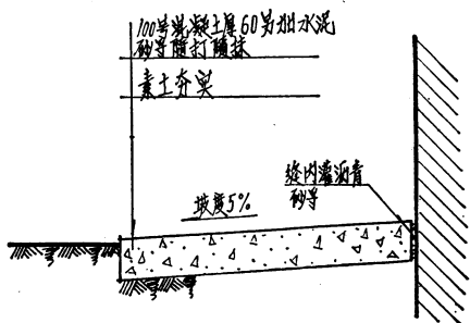
③ 混凝土散水
