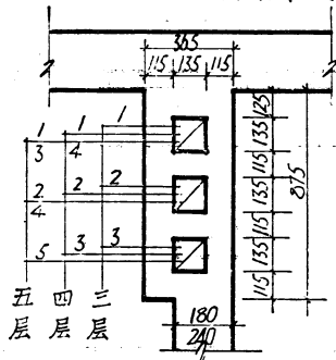
⑤ 三层楼单间
