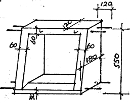
混凝土框示意
