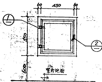
垃圾口铁门
