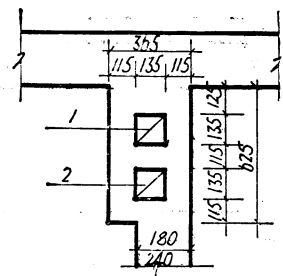
③ 二层楼单间
