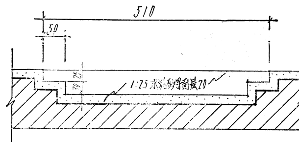
铁篦地槽剖面图
