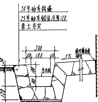
② 乱石砌散水
