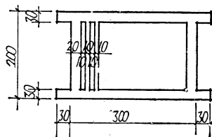
铸铁通风蓖
