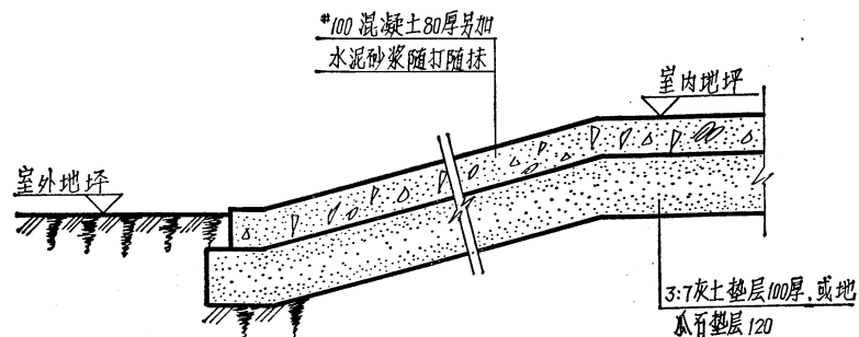
⑨ 混凝土坡道
