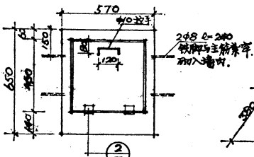
倾倒口立面
