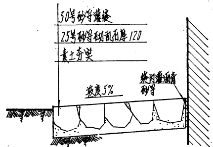
② 乱石砌散水
