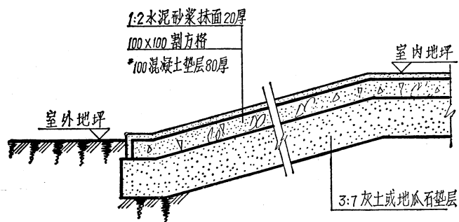
⑥ 混凝土坡道
