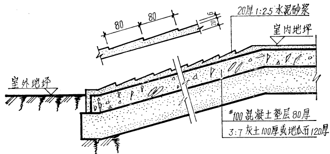
⑧ 混凝土防滑坡道
