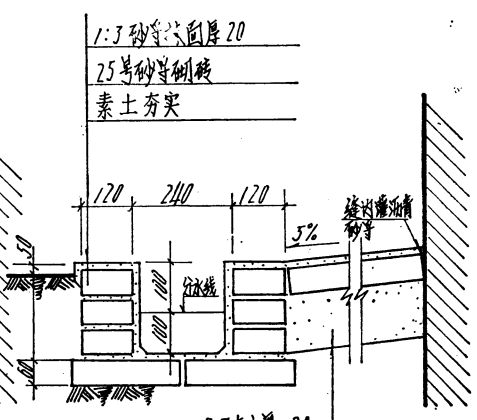
⑤ 砖砌明沟
