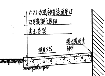
④ 混凝土散水
