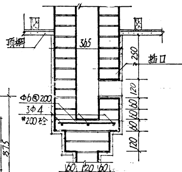
⑦ 120 墙挑烟囱剖面
