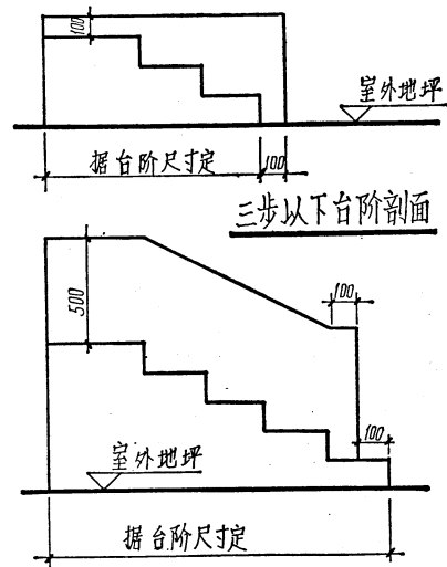
三步以上台阶剖面
