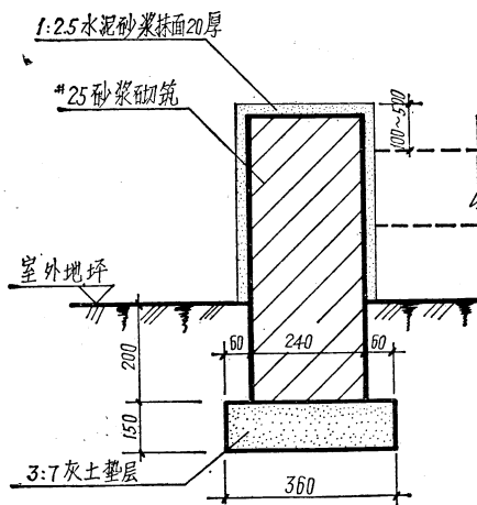
⑩ 砖砌台阶座
