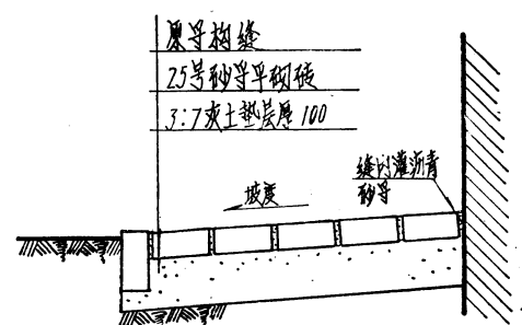
① 砖砌散水
