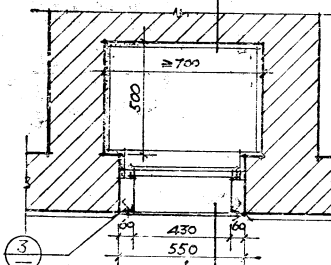
垃圾口平面
