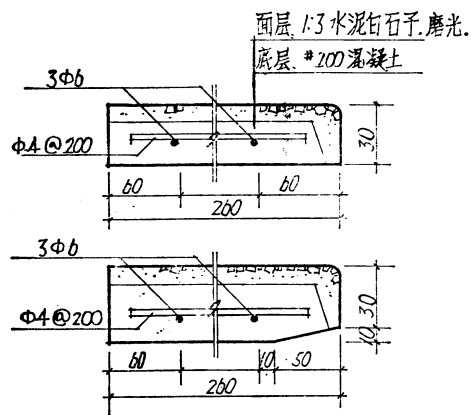
水磨石窗台板
