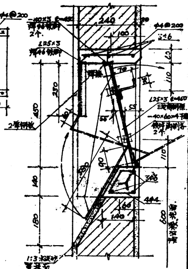
2-2 剖面
