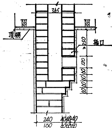
⑧ 180 墙挑烟囱剖面
