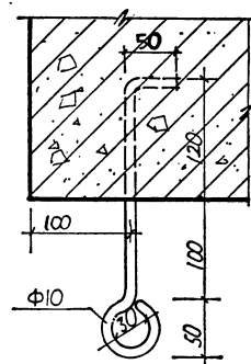
⑤ 吊钩〈在梁下或楼板下〉
