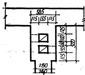
② 平房双间
