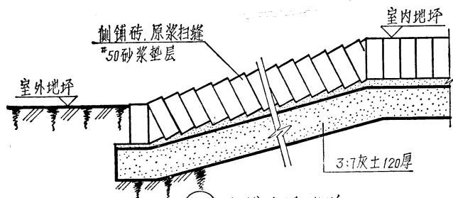
⑦ 砖铺防滑坡道
