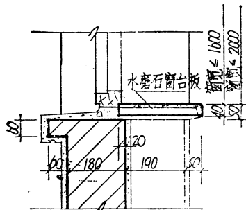
③ 有暖气槽
