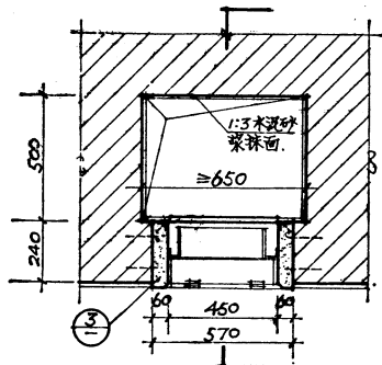
垃圾道倾倒口平面
