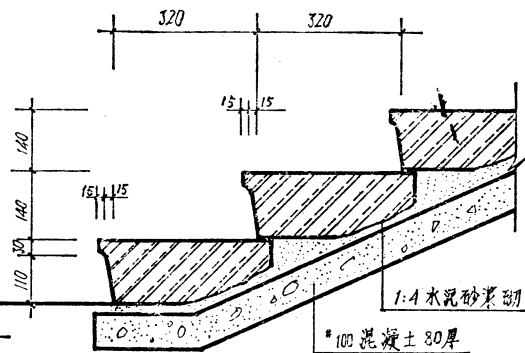
⑤ 剁斧石台阶
