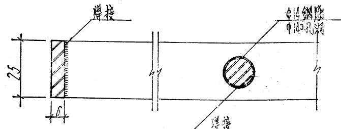
1-1 剖面图
