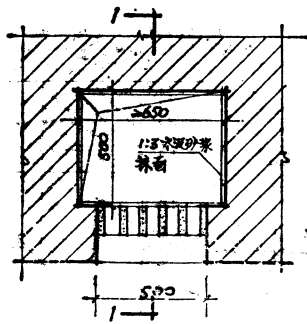
垃圾道通风洞平面
