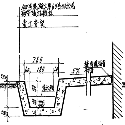
③ 混凝土散水
