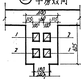
④ 二层楼双间
