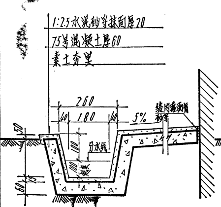
④ 混凝土散水
