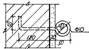
⑥ 吊钩 (在砖柱或砖墙上)
