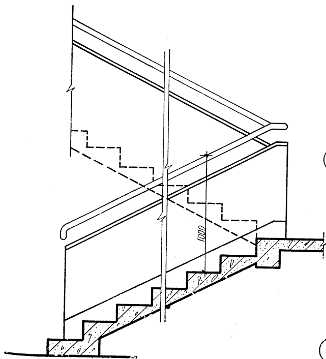
栏板扶手
