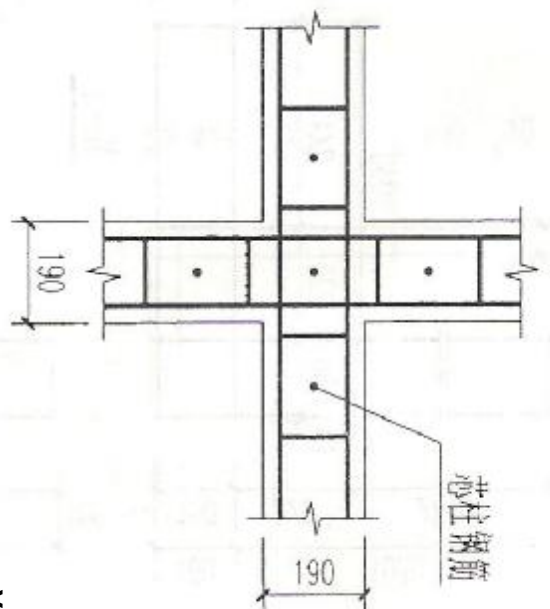
3 圈梁十字交接处平面
