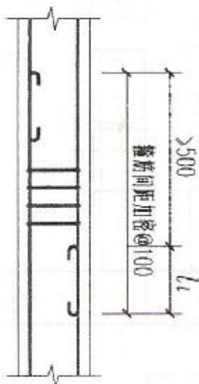
圈梁钢筋搭接
