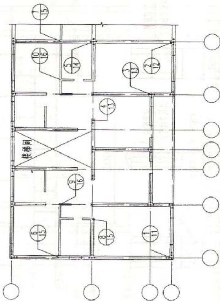
芯柱、墙体连接节点选用示例
