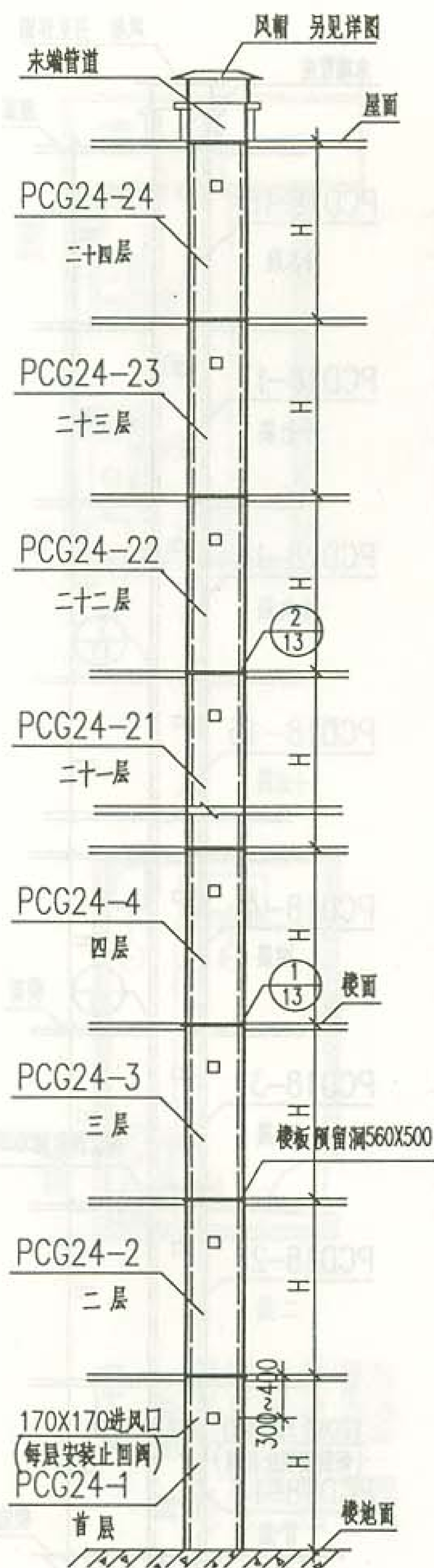
PCG24型系统组装图 (≤24层)
