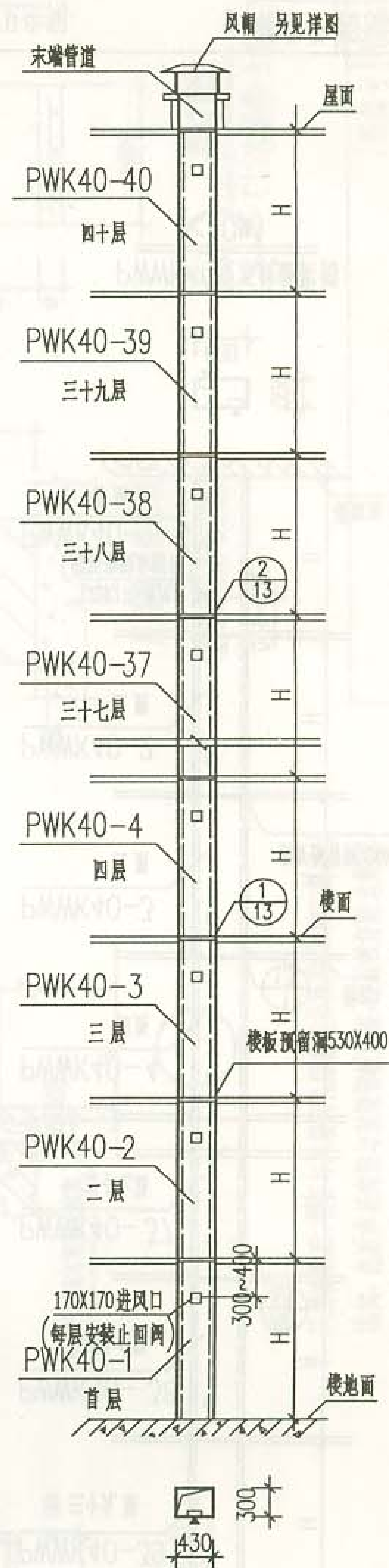
PWK40型系统组装图 (≤40层)
