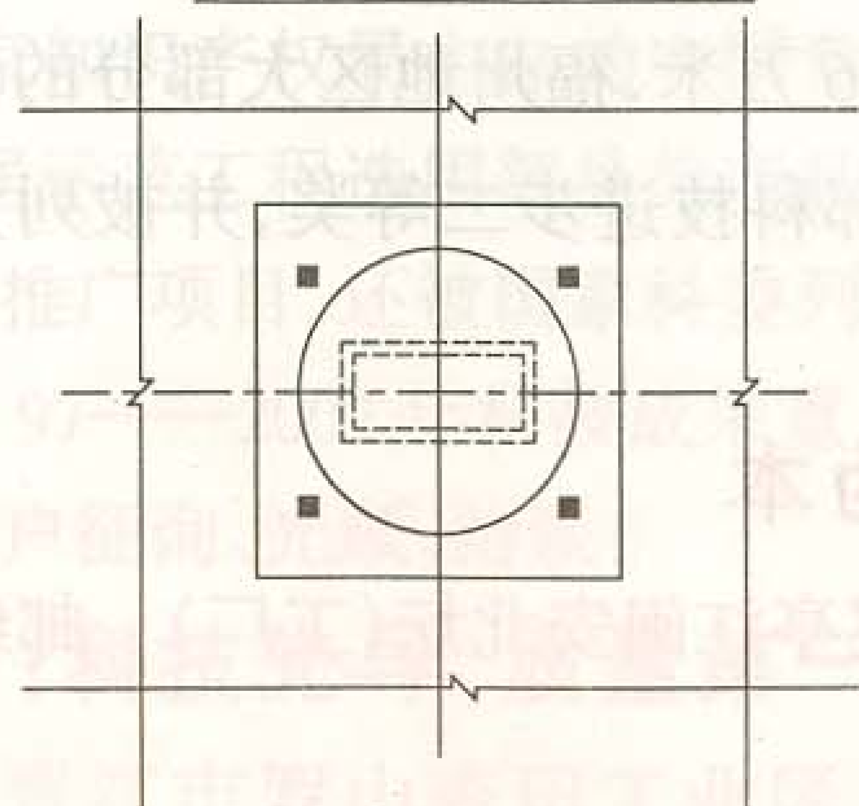
A-A 自力式风帽出屋面平面图
