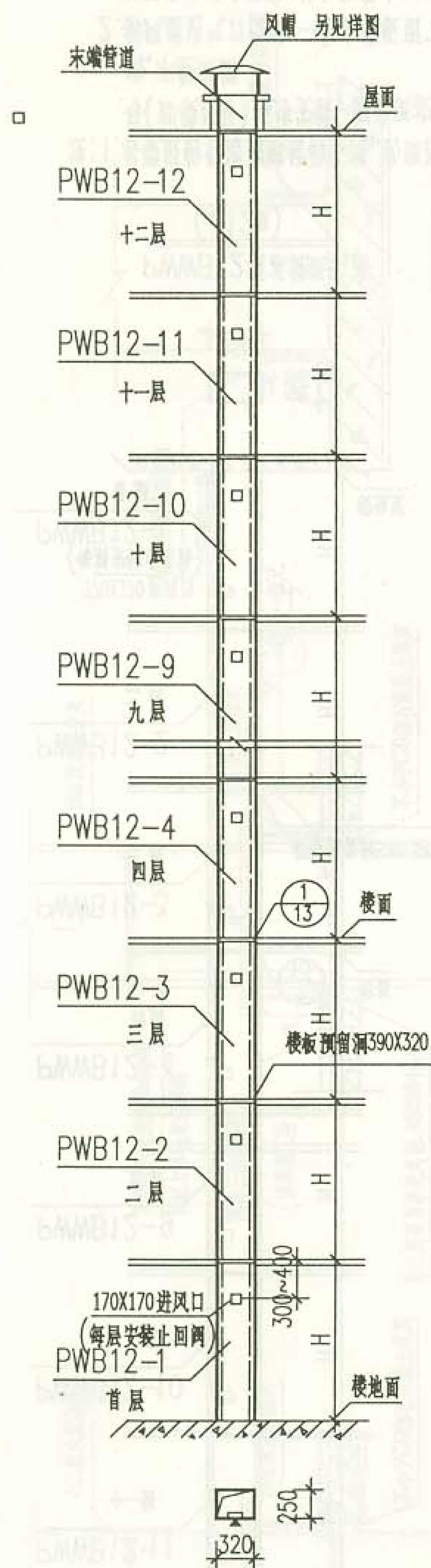
PWB12型系统组装图 (≤12层)
