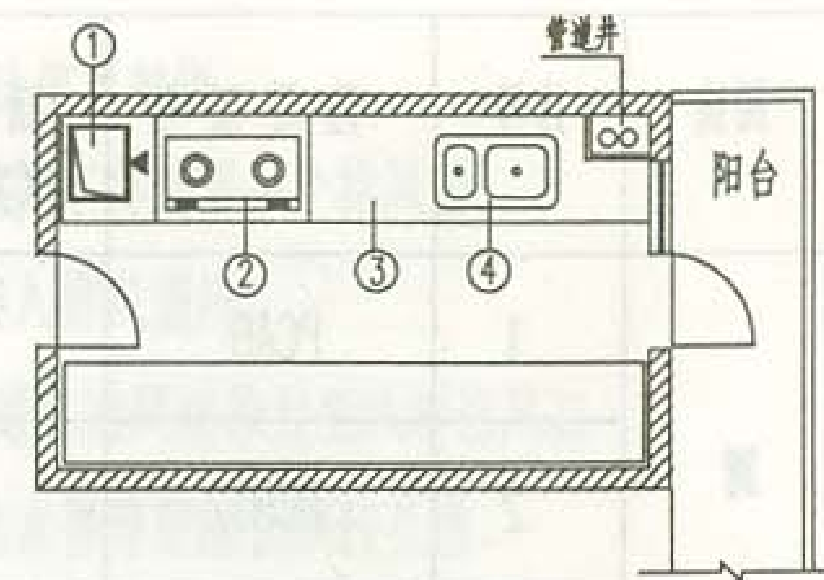
厨房平面布置示意图 (三)
