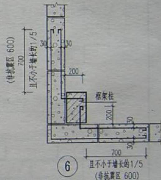
墙体与框架柱或混凝土墙拉结
