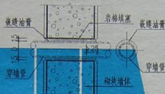
2 穿墙管做法
