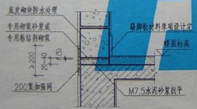
3 楼面部位构造
