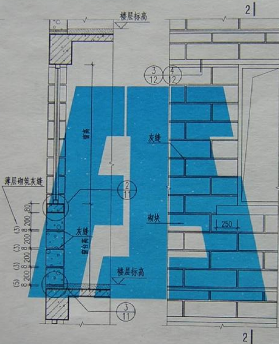
1-1剖面
