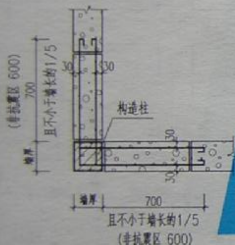
2 墙体与构造柱拉结
