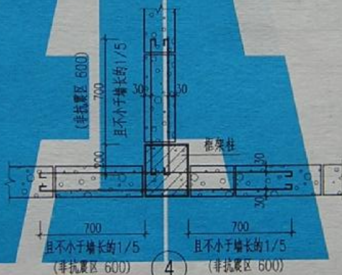
墙体与框架柱或混凝土墙拉结
