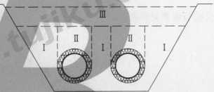
② 管道回填土部位划分示意图
