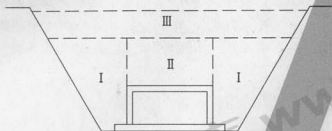
① 检查井回填土部位划分示意图
