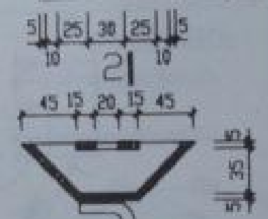
② 地轮
