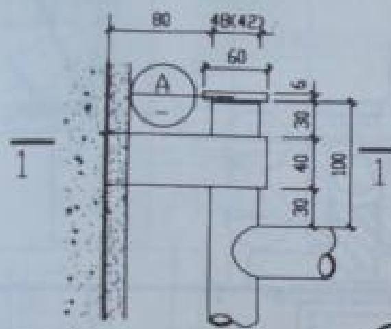
上轴立面
