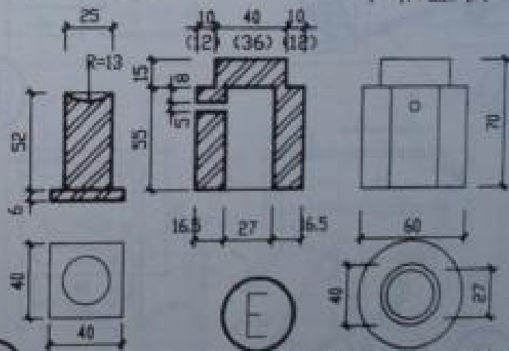
下轴立面
