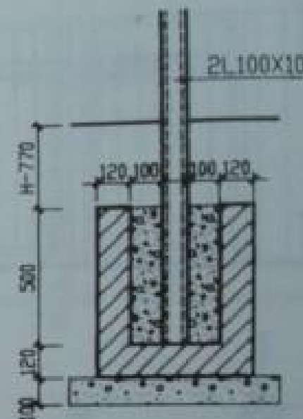
混凝土柱基础
