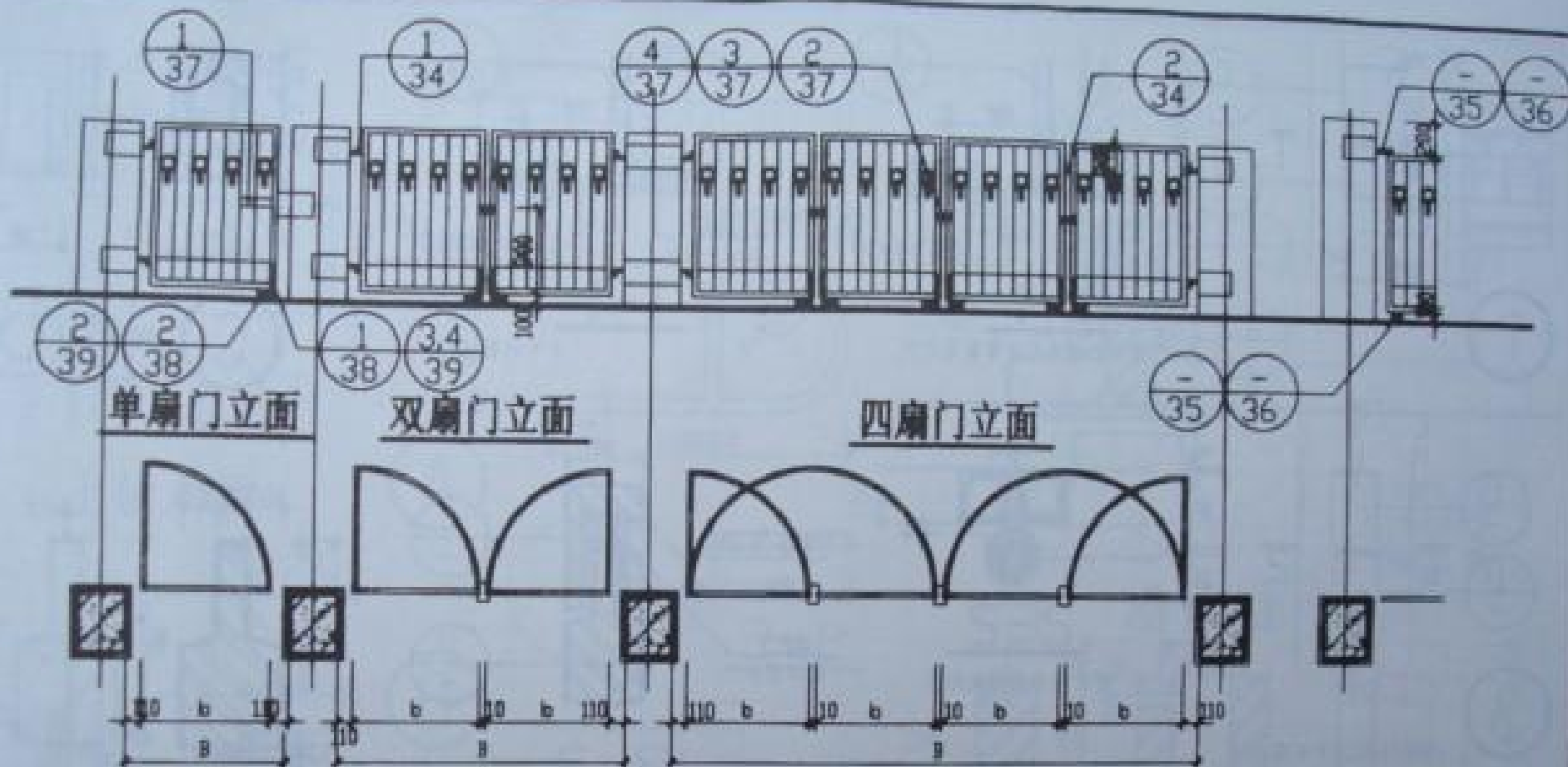
大门洞口宽度表
