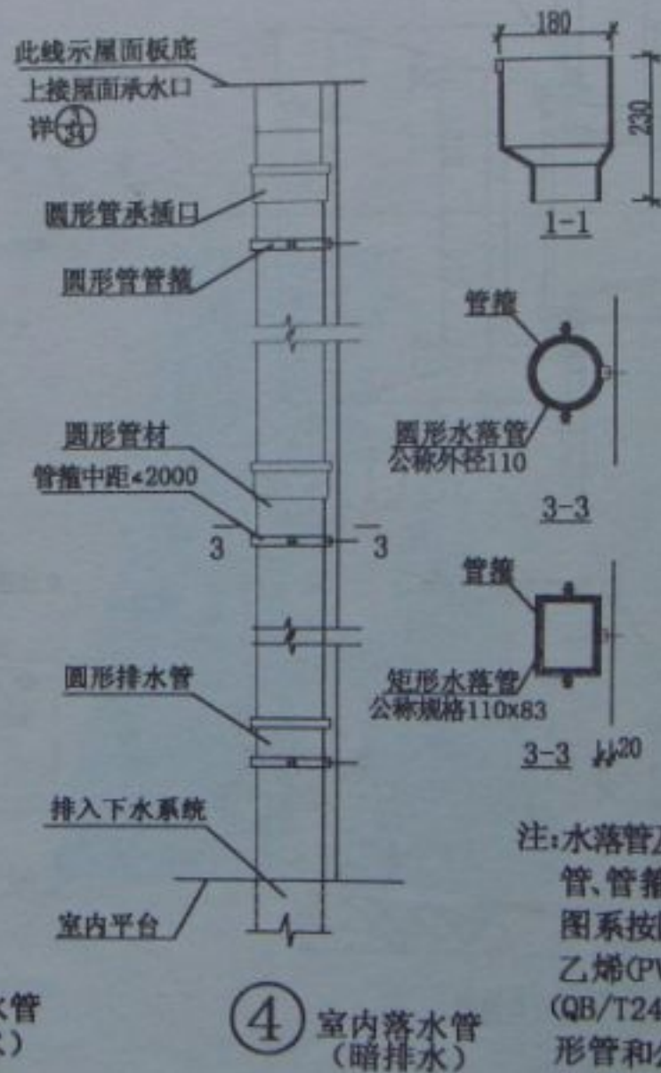
水落管及水斗大样
