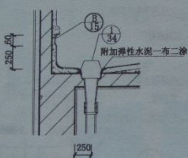
① (屋面无保温隔热层)
