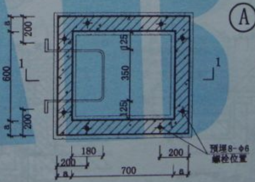
上屋面人孔平面图
