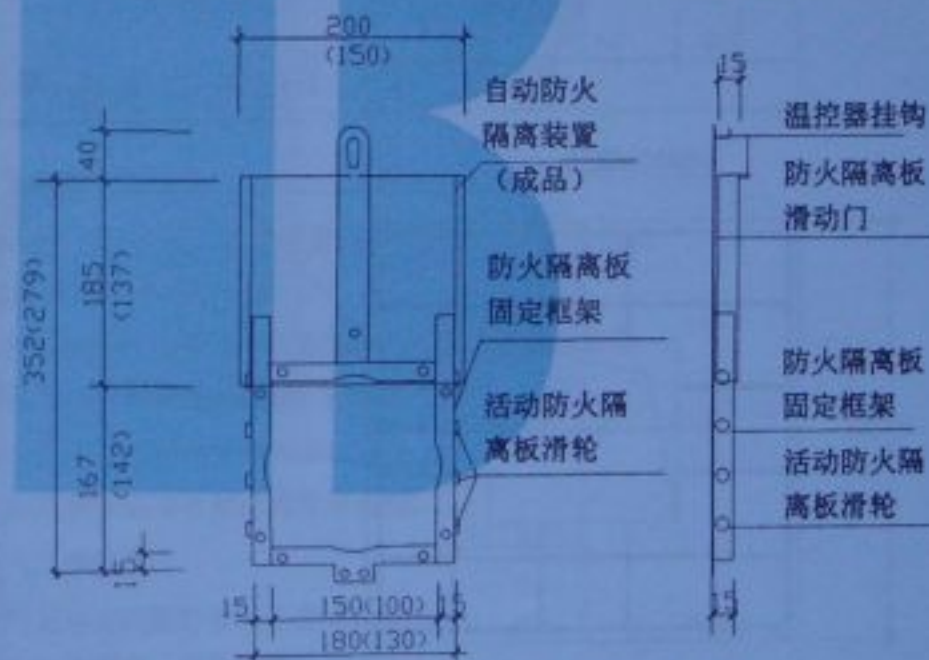
自动防火隔离装置立面侧面图
