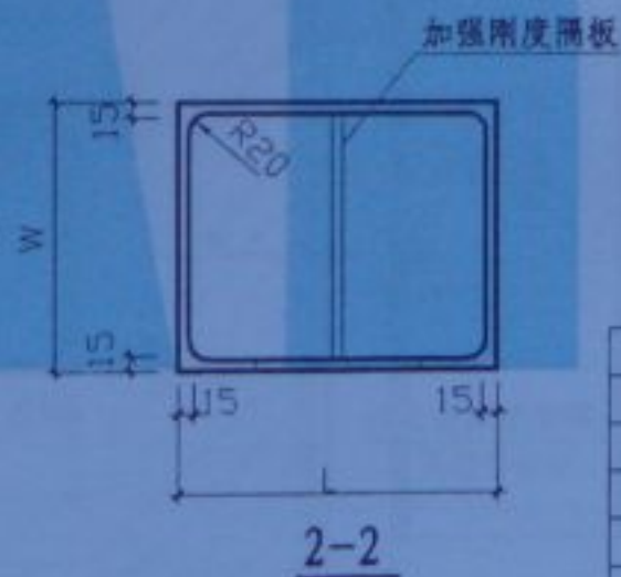
厨房止回阀连接底板 (成品)
