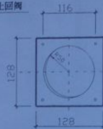
卫生间止回阀连接底板 (成品)
