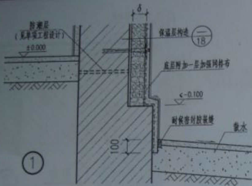
外墙勒脚1 (用于无地下室)
