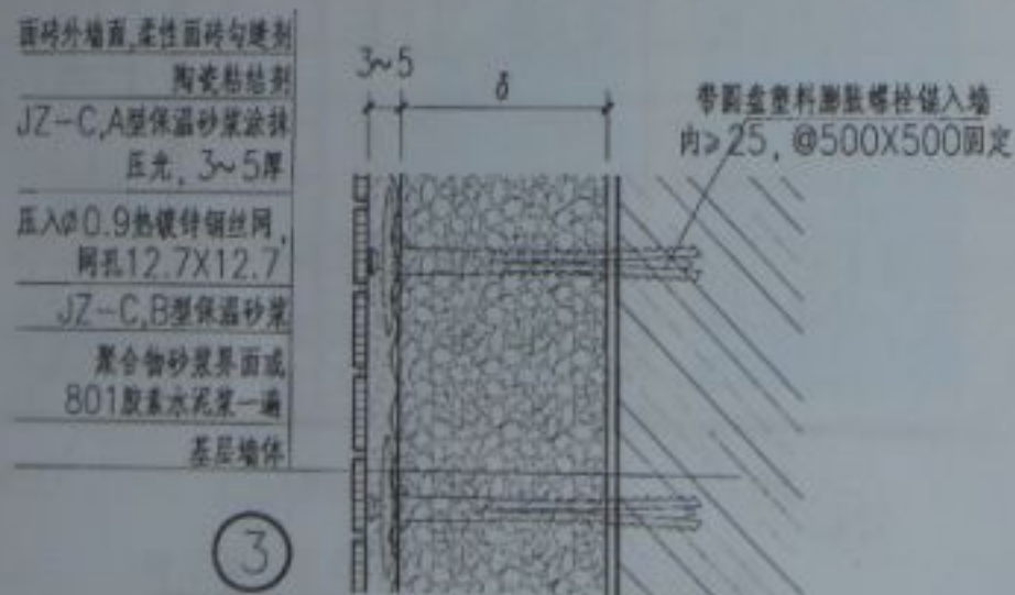
面砖外墙 (外墙3)
