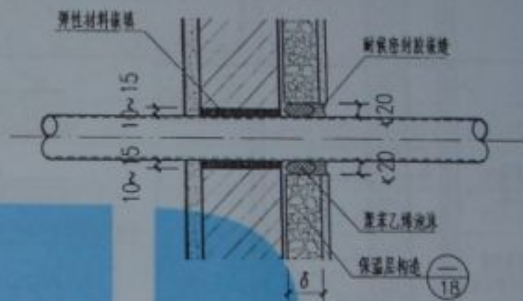
管道穿墙图
