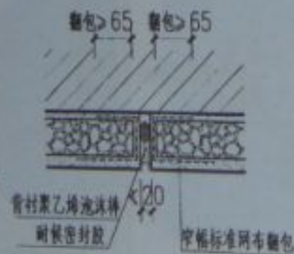
垂直系统变形缝
