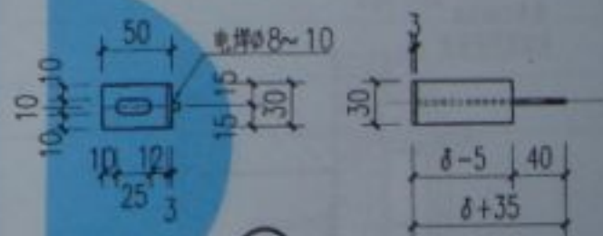
管箍固定件
