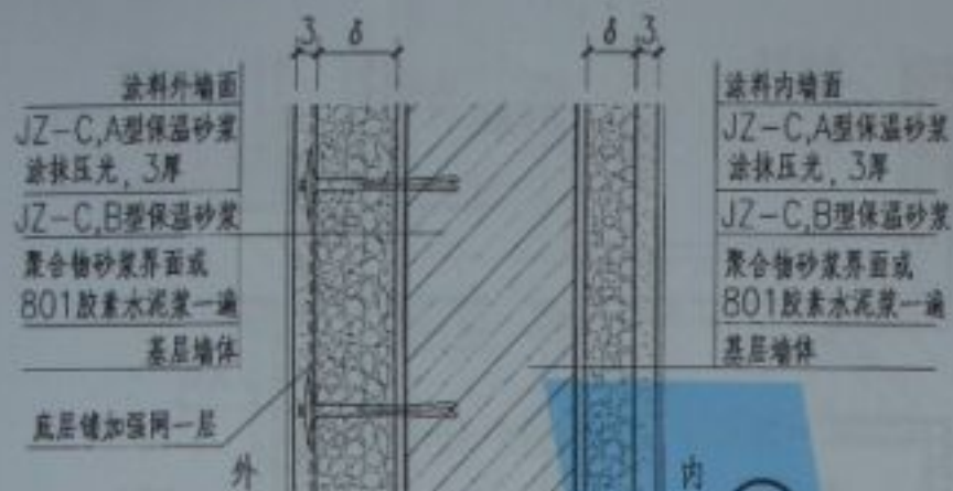
① 外墙内外面 (外墙4) (外保温层厚度 \delta < 30 )
