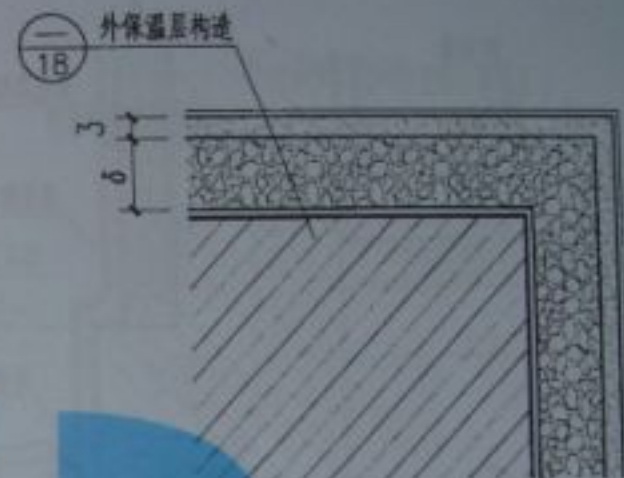
阳角 (用于二层及以上) ②
