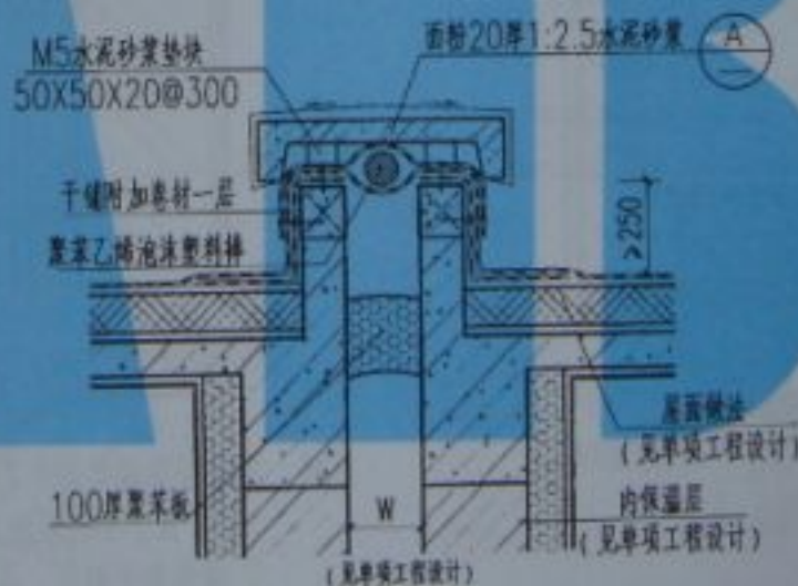
屋面变形缝2
