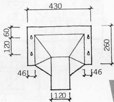
2 铸铁雨水口立面
