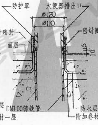
⑤ 座便安装图
