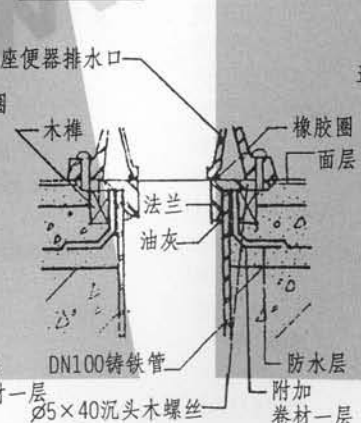
⑥ 座便安装图
