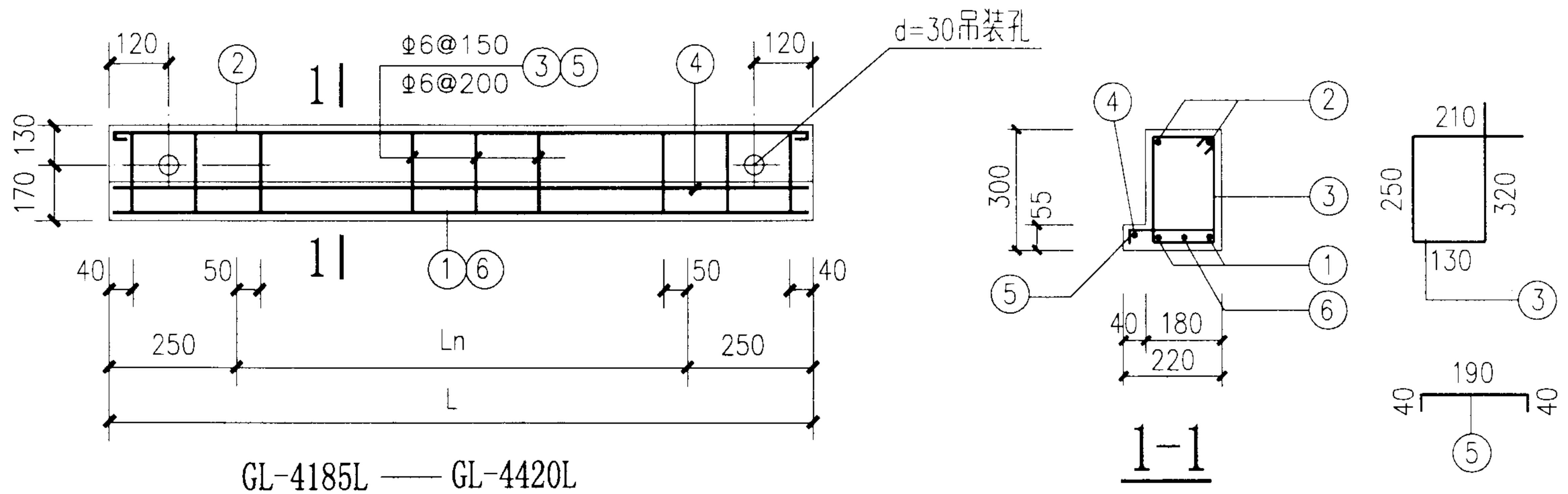
每一构件钢筋表
