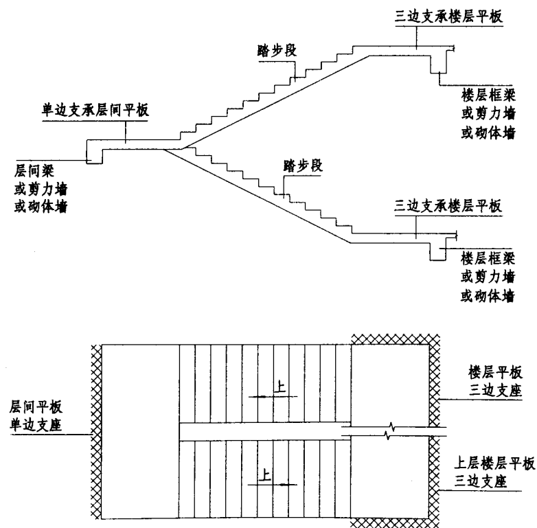
GT型（有层间和楼层平板的双跑楼梯）
