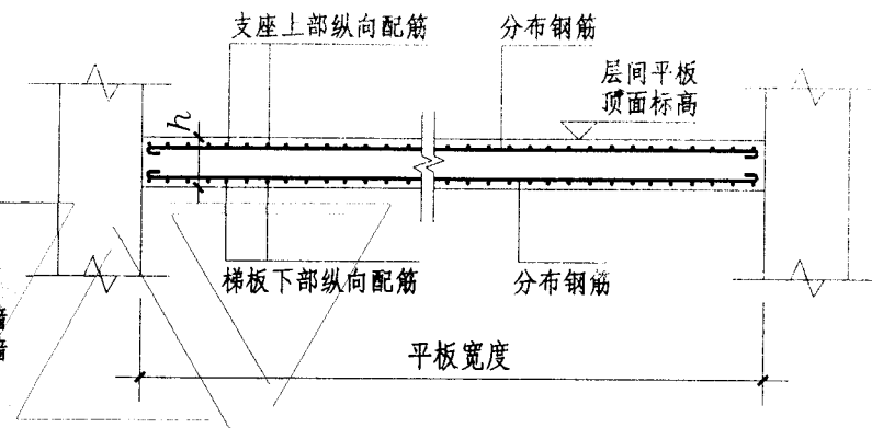
E-E 楼梯平板钢筋构造
