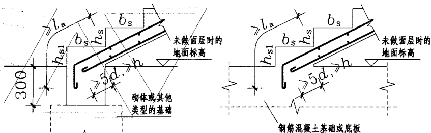
各型楼梯第一跑与基础连接构造
