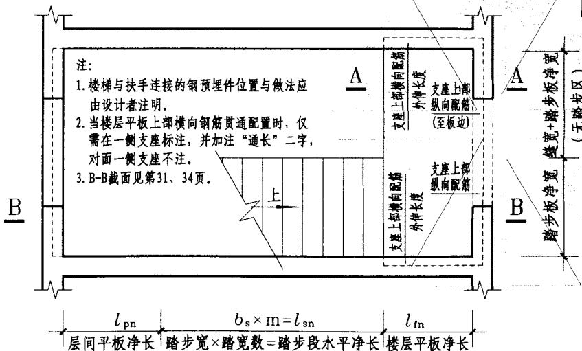
FT、GT最高一跑楼层平板注写方式与配筋构造
