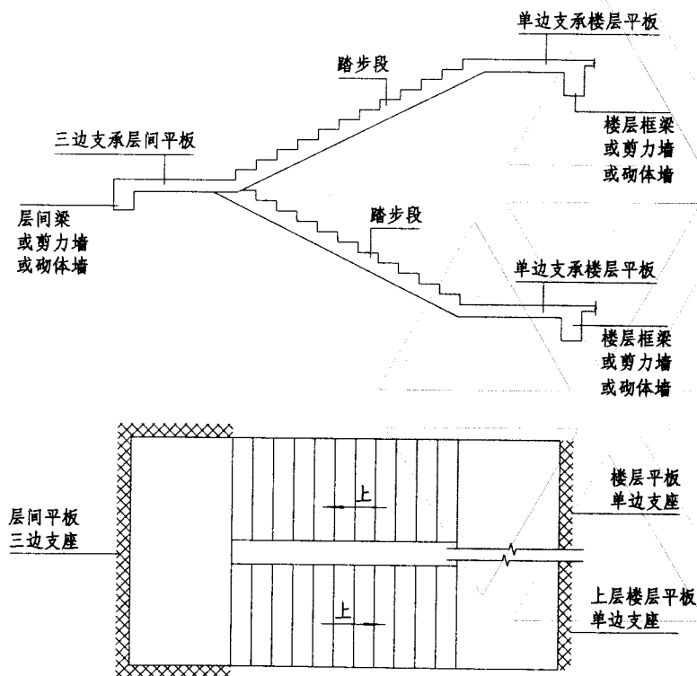
HT型（有层间和楼层平板的双跑楼梯）
