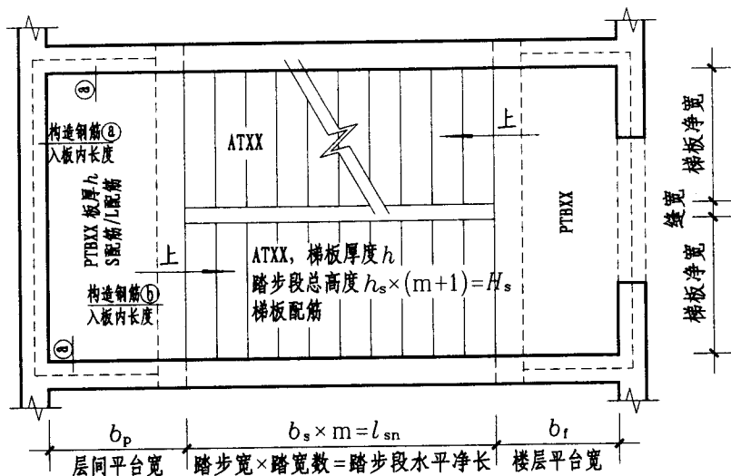
图1. 注写方式 标高XXX—标高XXX楼梯平面图 注: 楼层、层间平台板 梯板分布钢筋: XXXXXX PTB注写方式与构造详见第48页。 平台板分布钢筋: XXXXXX
