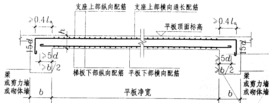
D-D 楼梯平板钢筋构造
