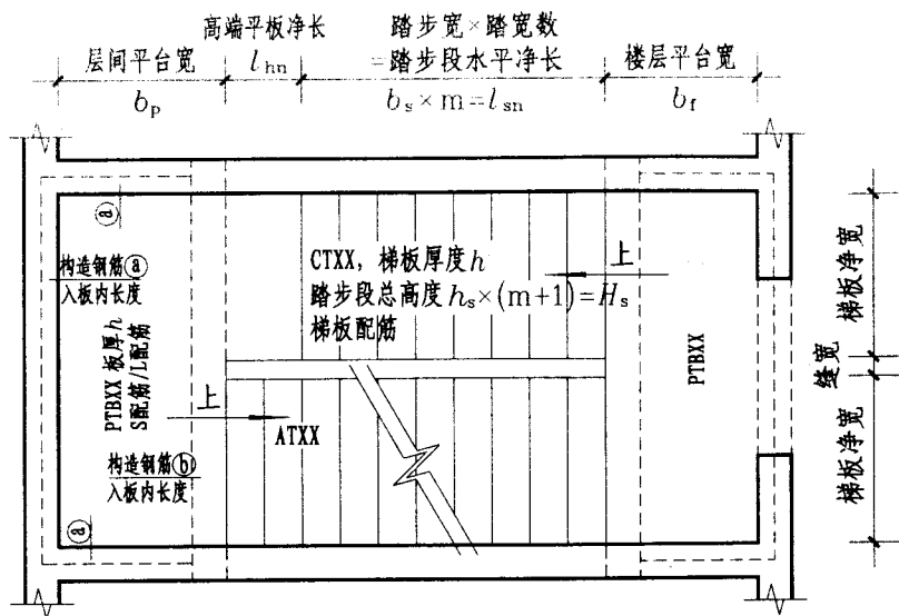
图1. 注写方式 标高XXX—标高XXX楼梯平面图 注: 楼层、层间平台板 梯板分布钢筋: XXXXXX 平台板分布钢筋: XXXXXX 构造详见第48页。
