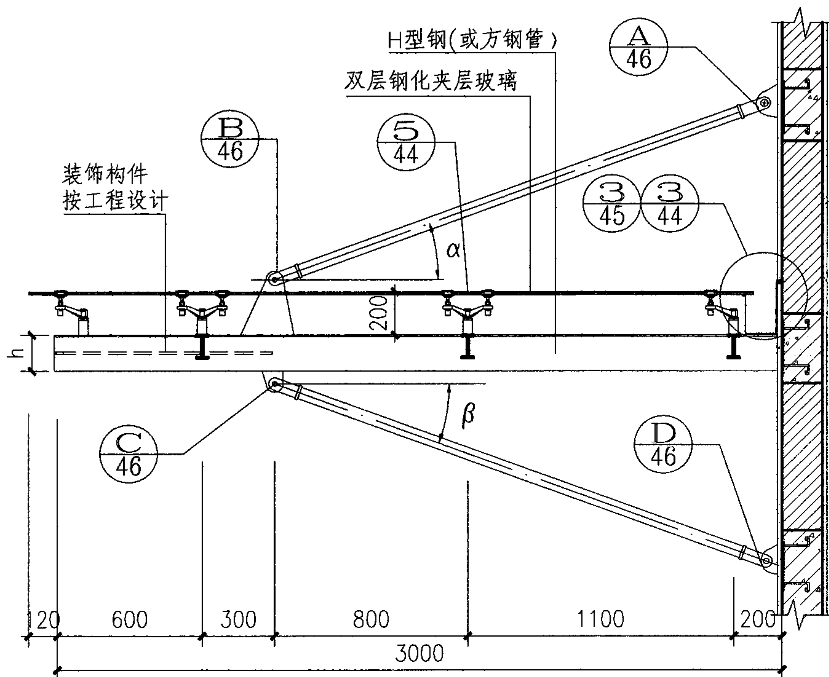
1-1剖面
