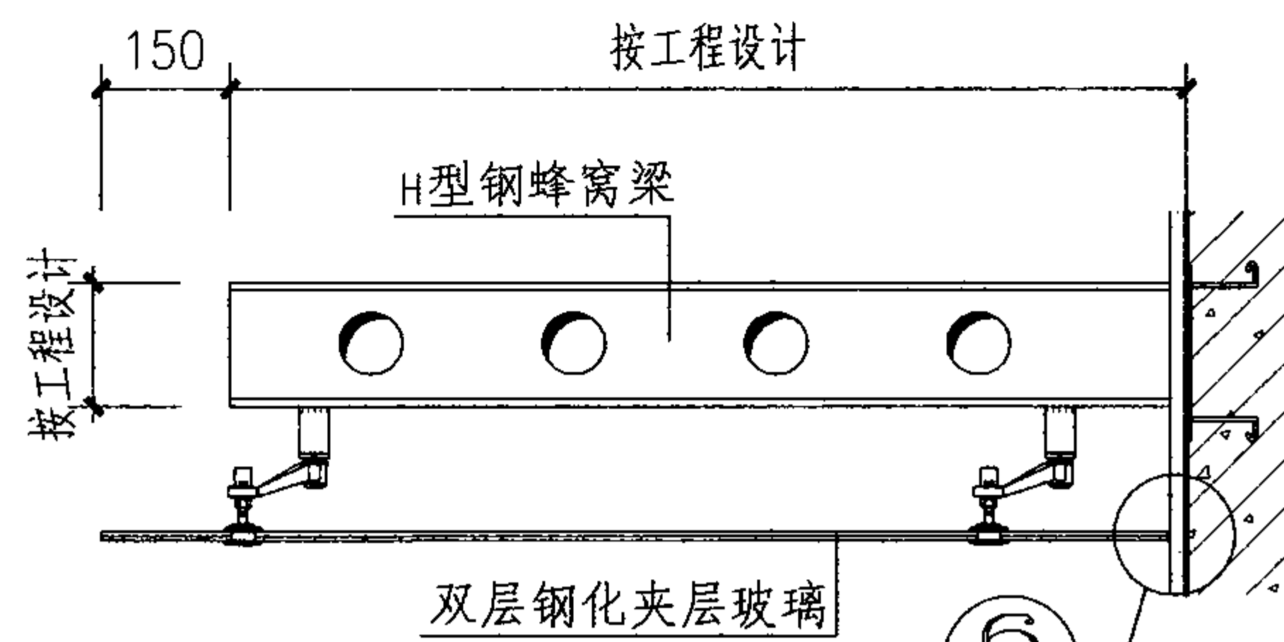
2-2剖面
