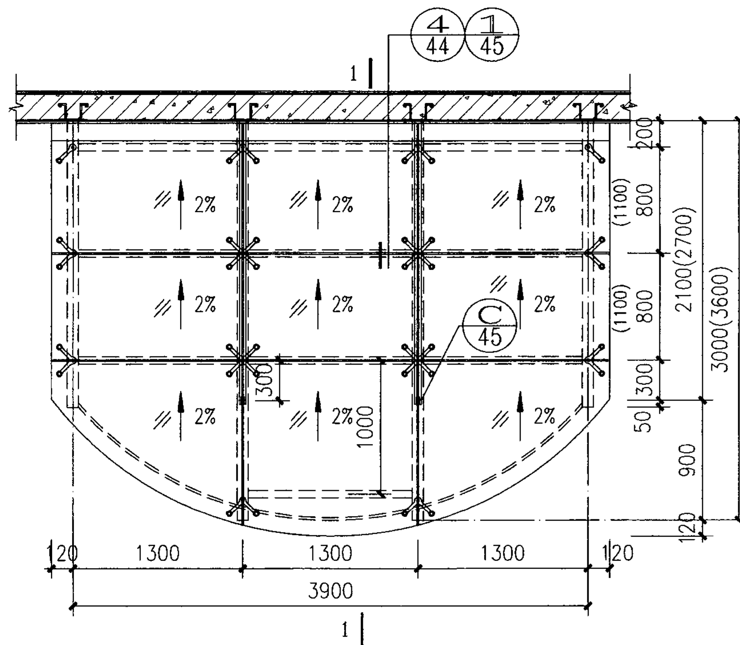
平面 (点支承)
