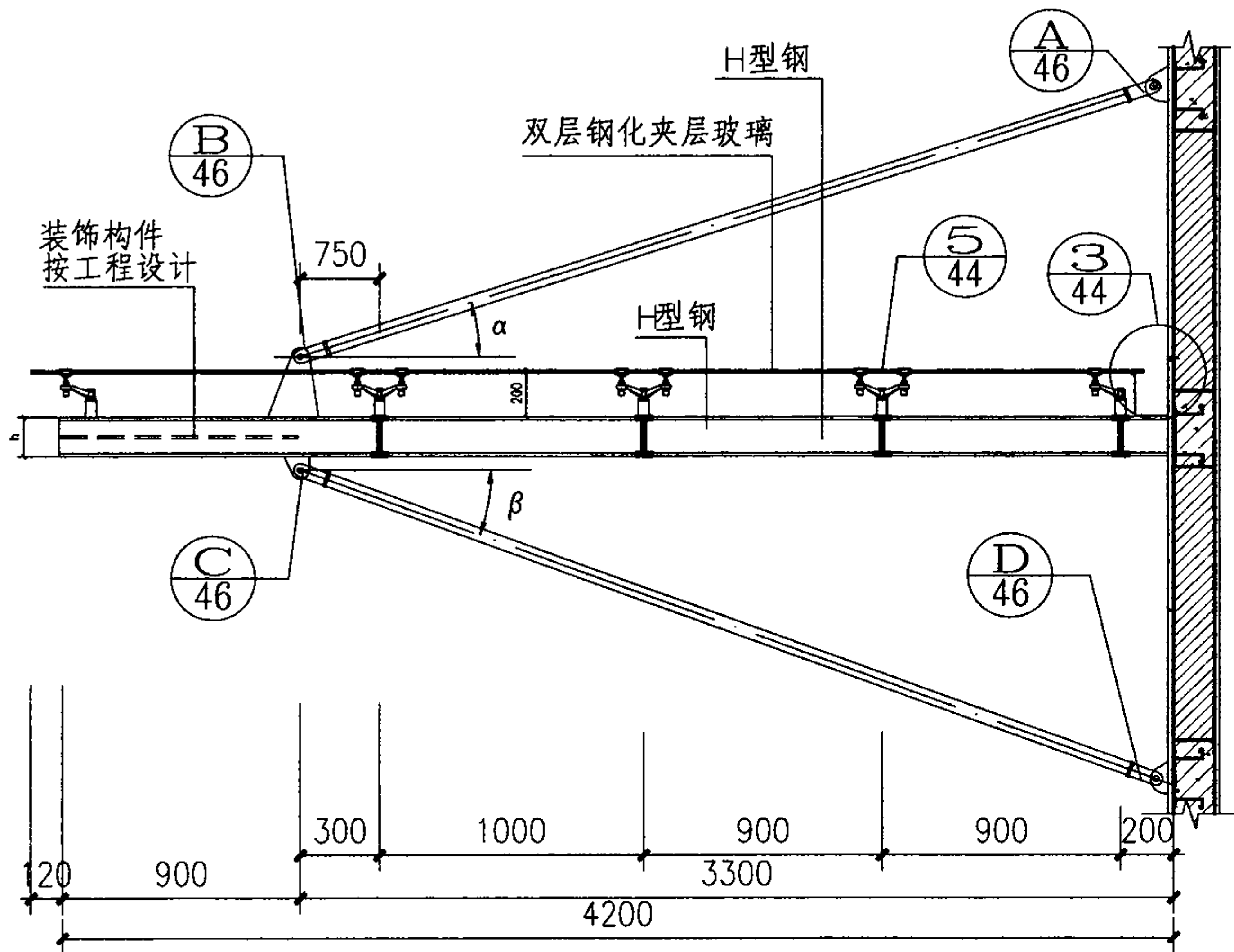
1-1剖面
