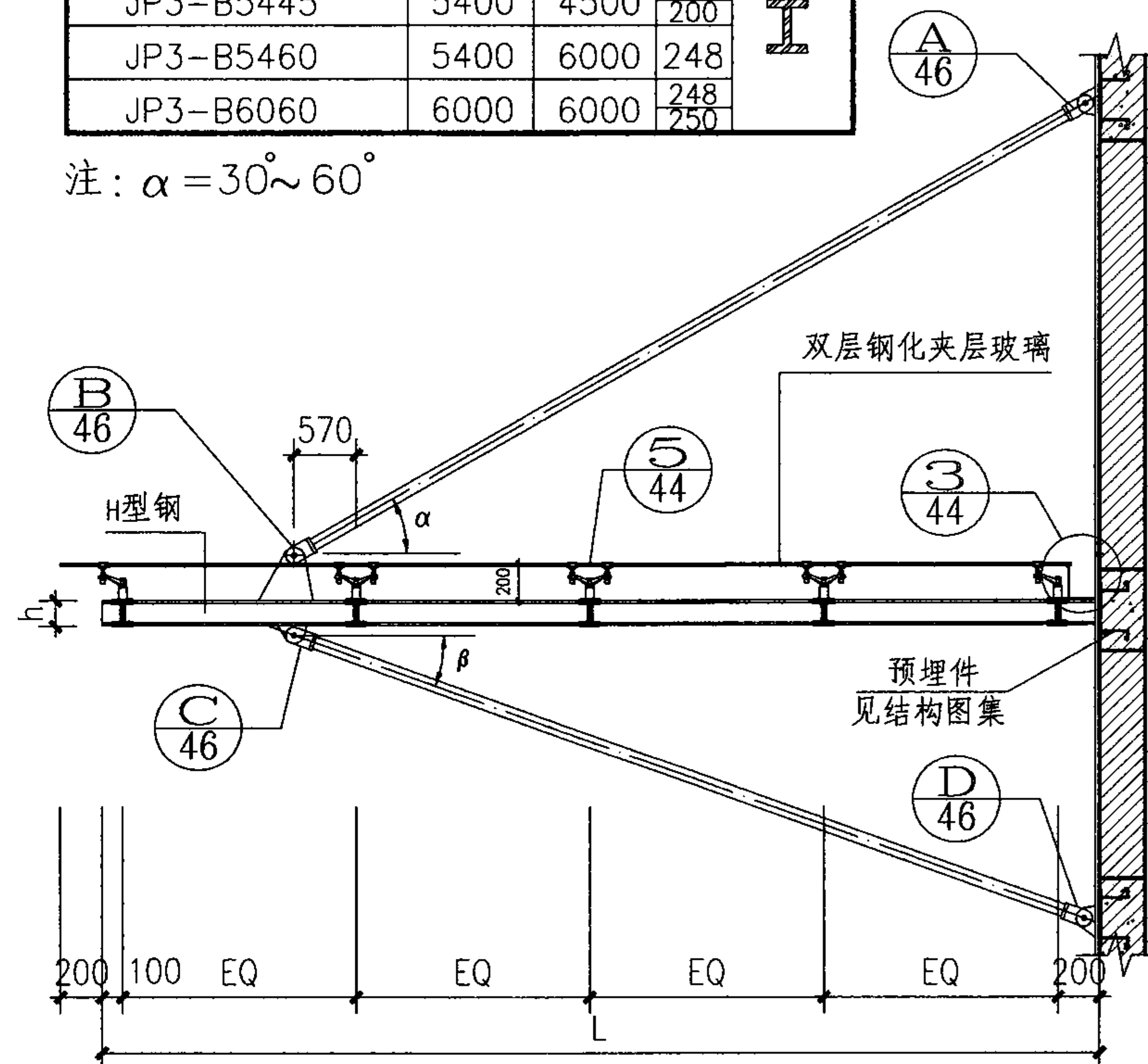
1-1剖面
