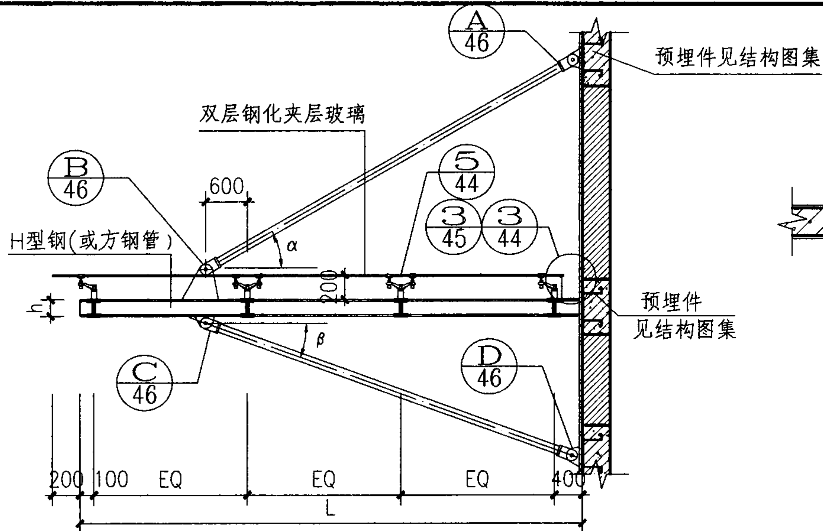
1-1剖面
