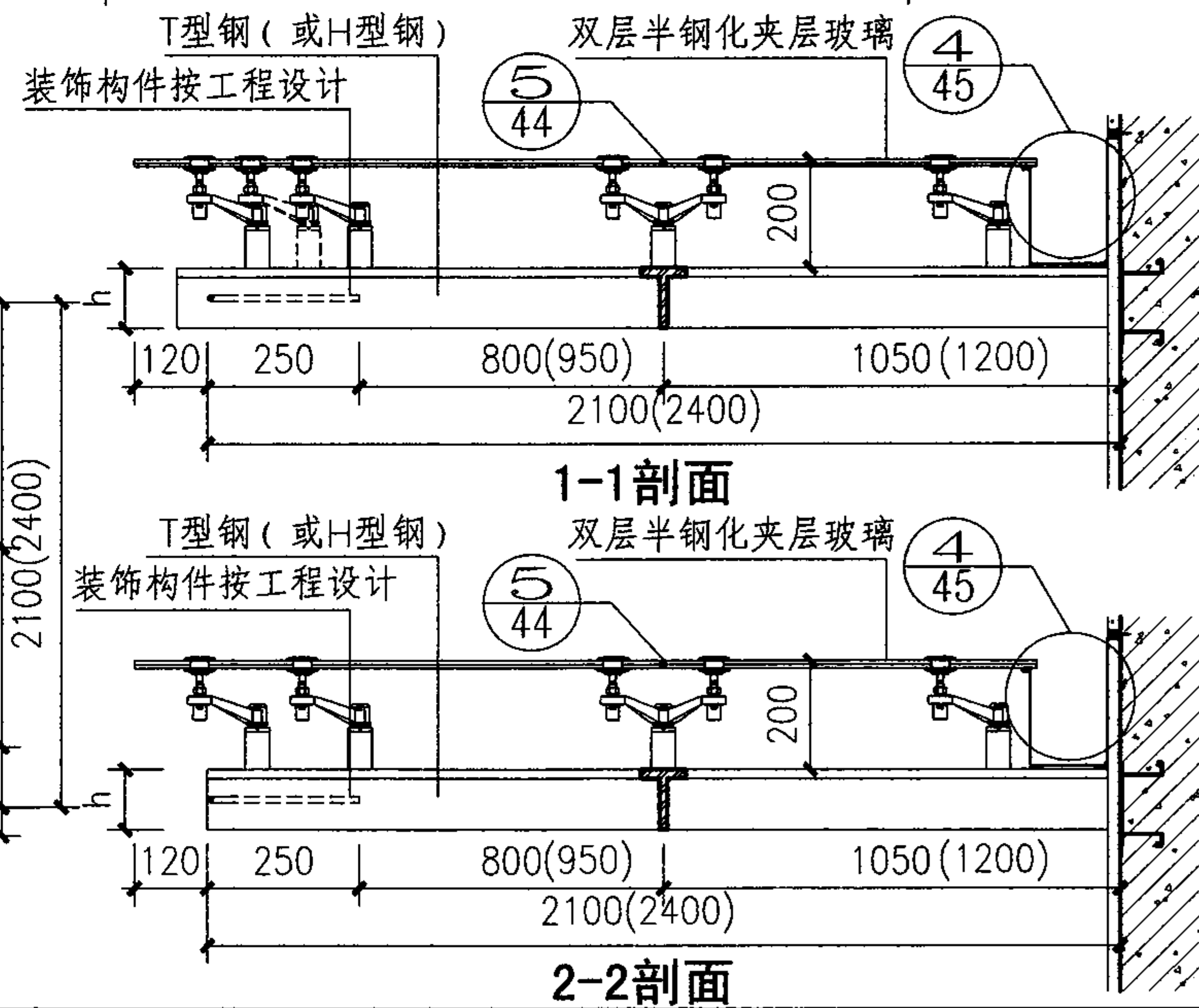
SP1-A21XX、A24XX 型钢雨篷 SP1-B21XX、B24XX 型钢雨篷
