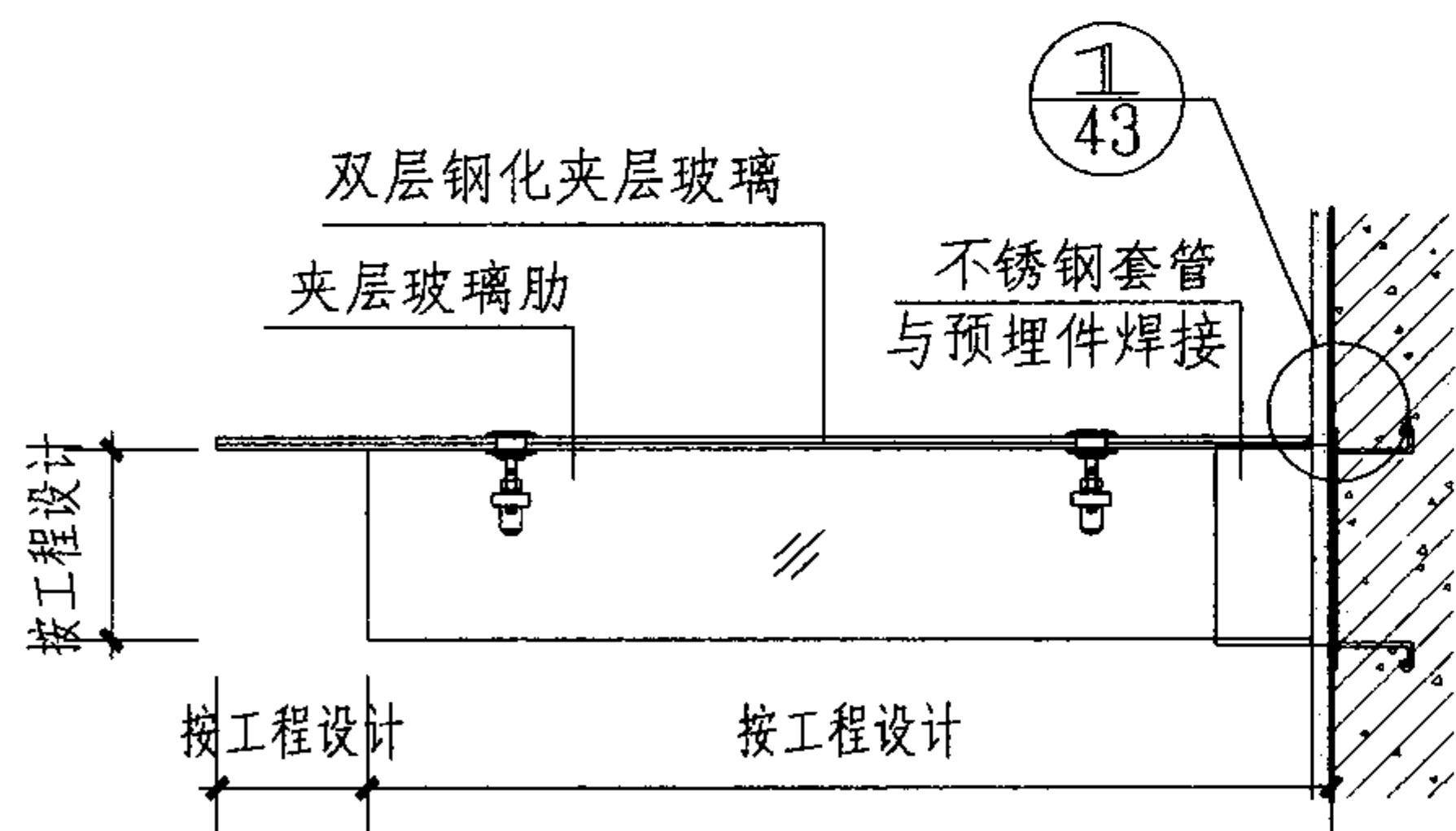
1-1剖面
