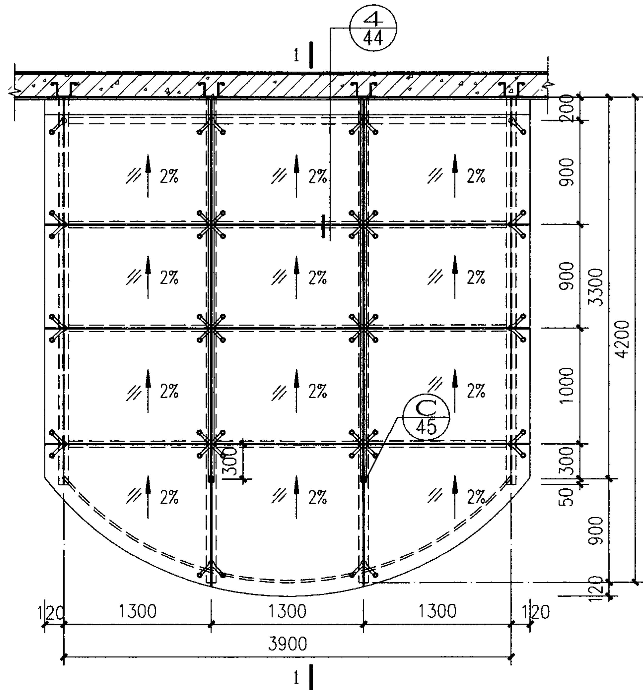
平面 (点支承)
