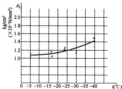
图 3 冰块的抗拉强度极限值试验曲线
