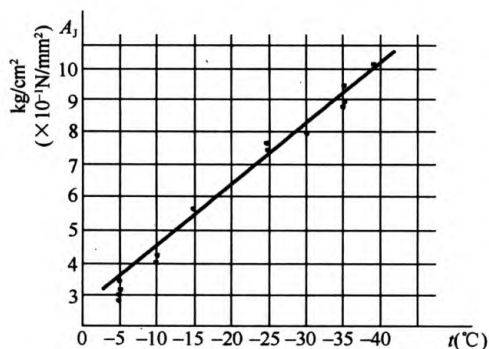
图 2 冰块的抗剪强度极限值试验曲线
