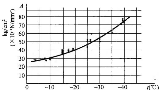
图 1 冰块的抗压强度极限值试验曲线
