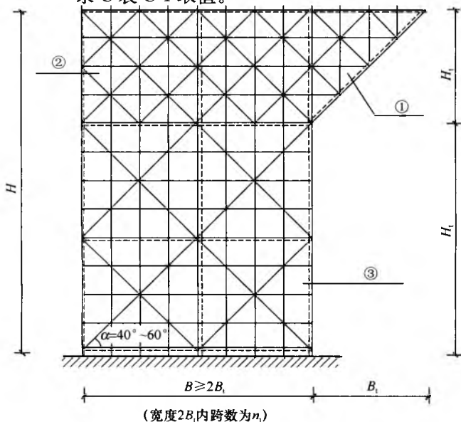
(a) 侧立面图
