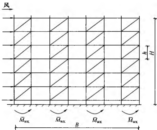
图 13 风荷载作用于支撑结构引起单元桁架的整体弯矩图
