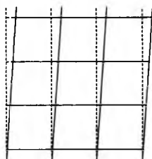
图 2 无剪刀撑框架式支撑结构的失稳模态图
