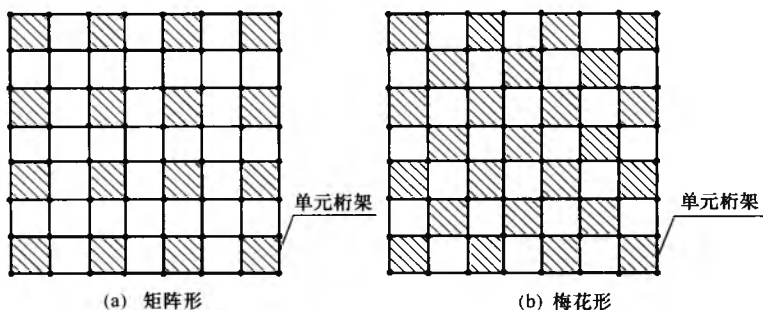
图 5.3.2 单元桁架组合方式布置平面图
