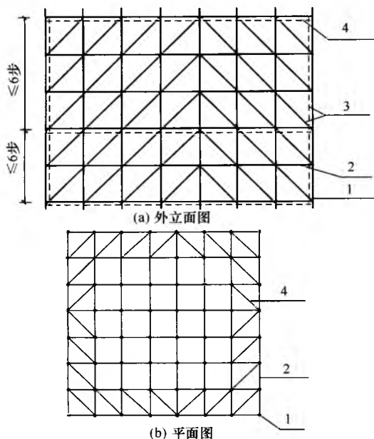
图 5.3.3 桁架式支撑结构斜杆布置图
