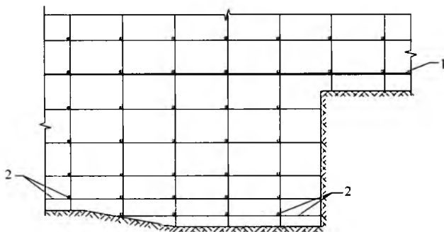
图 5.1.7 不同标高扫地杆布置图
