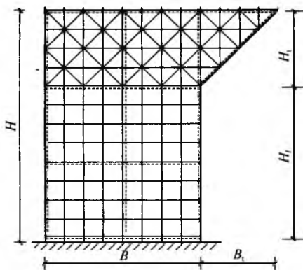
图 6.1.4 悬挑支撑结构剖面图 (1-1)
