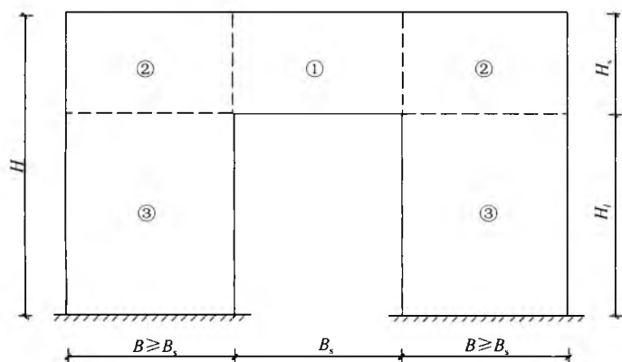
图 16 跨空支撑结构分区图
