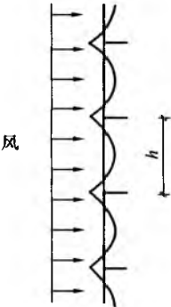
图 10 立杆节间局部弯矩立面图 这两种支撑结构应计算风荷载直接作用于立杆引起的立杆节间局部弯矩，如图 10
