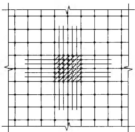
图 5.2.6 支撑结构加密区立杆布置平面图
