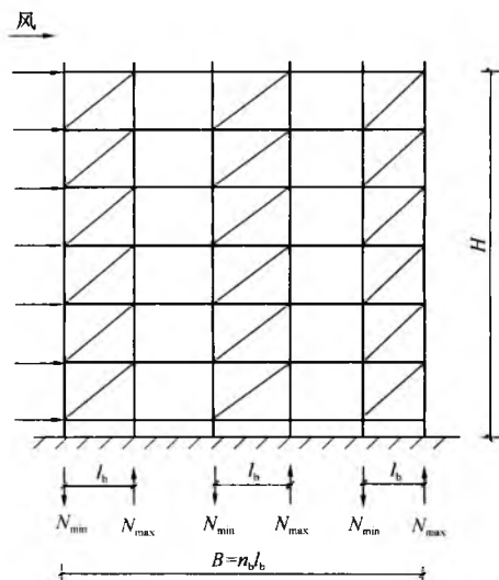
图 8 桁架式支撑结构（矩阵形）风荷载引起的立杆轴力图
