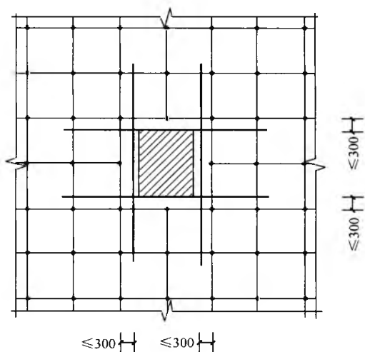
图 5.1.6 抱柱连接措施
