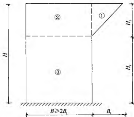
图 15 悬挑支撑结构分区图
