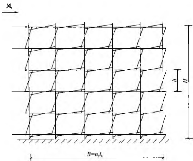
图 11 风荷载作用于无剪刀撑框架式支撑结构引起的立杆弯矩图
