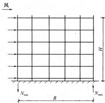
图 7 无剪刀撑框架式支撑结构风荷载引起的立杆轴力图
