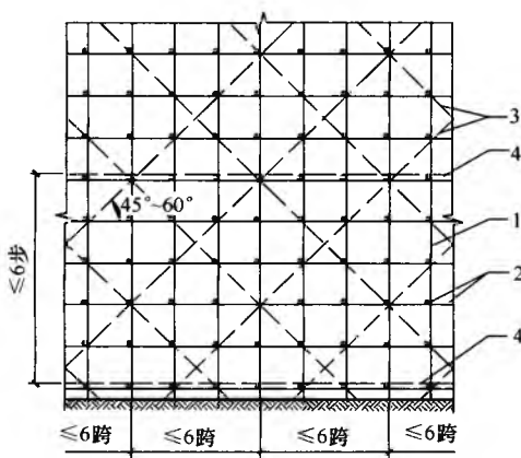
(b) 立面图
