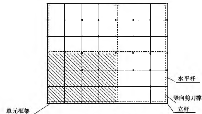
图 1 单元框架平面示意图
