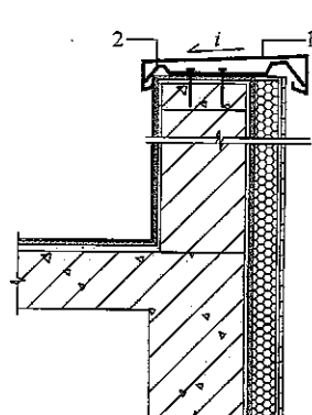
图 5.3.6-2 金属压顶女儿墙防水构造
