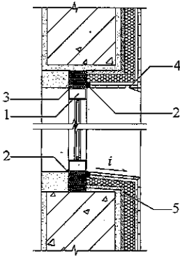
图 5.3.1-2 门窗框防水立剖面构造
