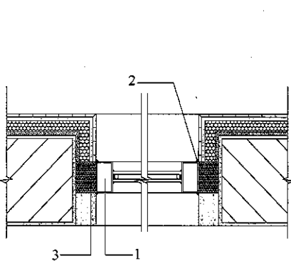
图 5.3.1-1 门窗框防水水平剖面构造
