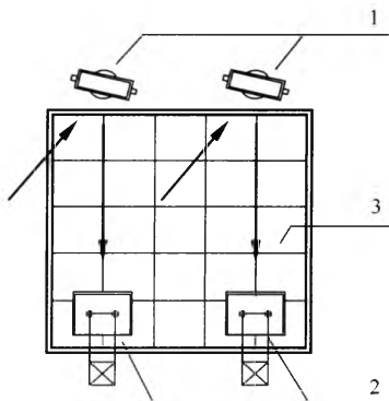
图1 建筑采光追逐镜平面示意
