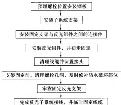
图 A.0.2 反光子系统安装工艺流程
