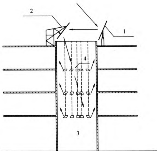
图 2 建筑采光追逐镜剖面示意
