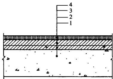
图 4.3.3 聚合物（树脂）防滑地面构造
