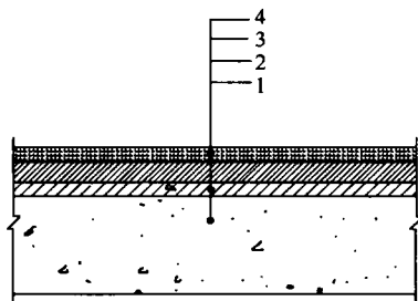
图 4.3.4 板块材料防滑地面构造
