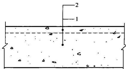
图 4.3.1 水泥混凝土防滑地面构造
