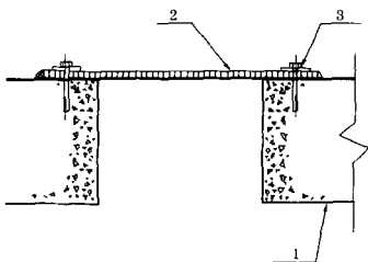
附图 8 防火板构造示意
