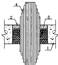
图4 电缆束穿越贯穿孔口的防火封堵示意
